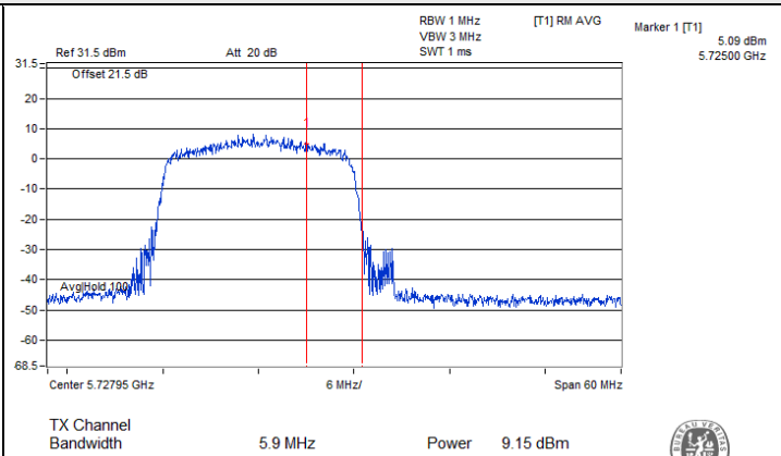
802.11ac (VHT20) CDD / Chain 1 : CH 144 (U-NII-3)
