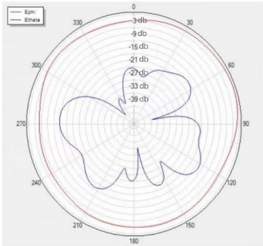
Theta=90 freq=2400MHz
