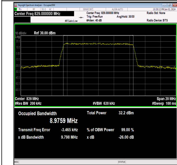
26(824-849)-10MHz-QPSK-26840-50RB#0-PASS
