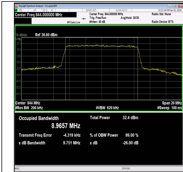
26(824-849)-10MHz-QPSK-26990-50RB#0-PASS
