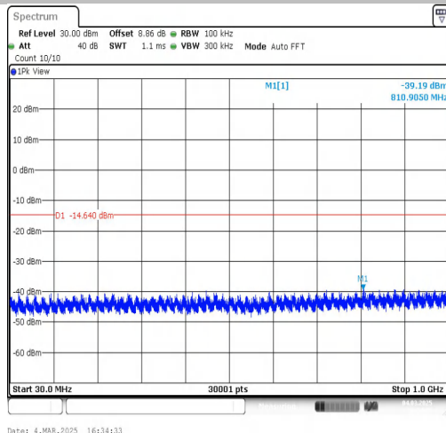
BLE_2M-Ant1-2402-30~1000-PASS
