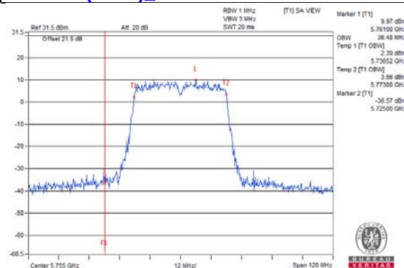
802.11ax (HE40) Chain 5 / CH151
