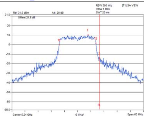
802.11a_Chain 6 / CH48
