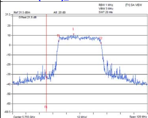
802.11ax (HE40) Chain 6 / CH151
