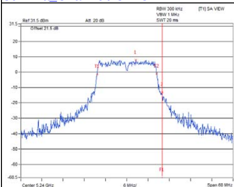
802.11a_Chain 6 / CH48
