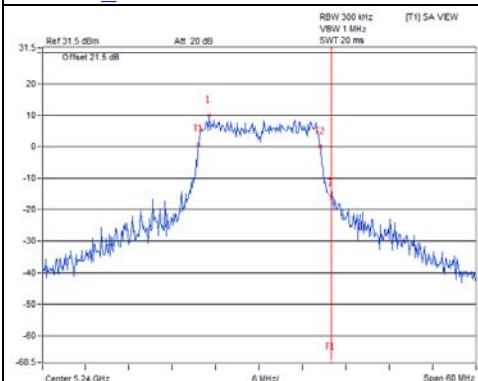
802.11a_Chain 4 / CH48
