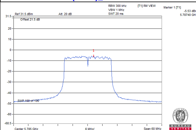
802.11ax (HE20)_Chain 2 / CH157
