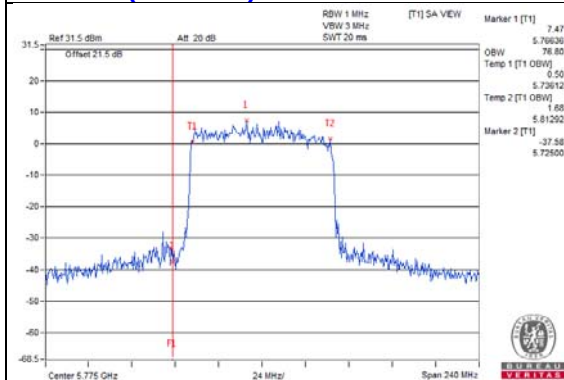
802.11ax (HE80+80) / Chain 6 : CH155
