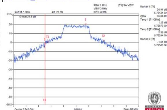
802.11ax (VHT20)_Chain1 / CH149
