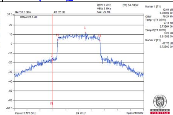
802.11ax (VHT80)_Chain1 / CH155
