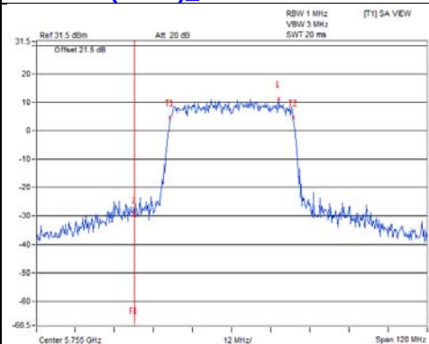
802.11ax (HE40) Chain 4 / CH151
