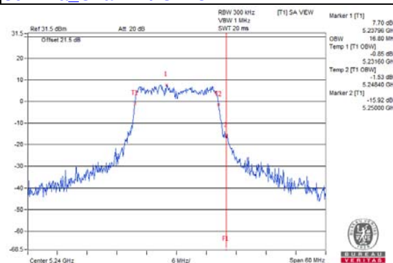
802.11a_Chain 7 / CH48
