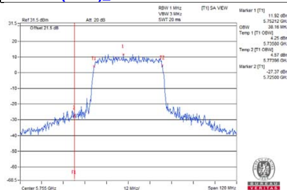
802.11ax (HE40) Chain 7 / CH151
