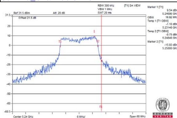
802.11a_Chain 7 / CH48
