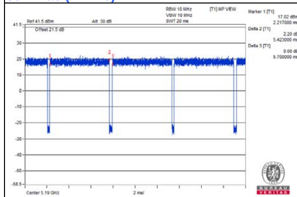
802.11ac (VHT80+80)
