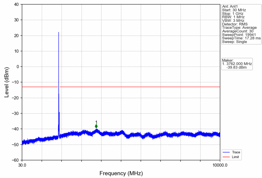
Band2_20MHz_16QAM_MCH_1880MHz_RB_1_0_NTNV
