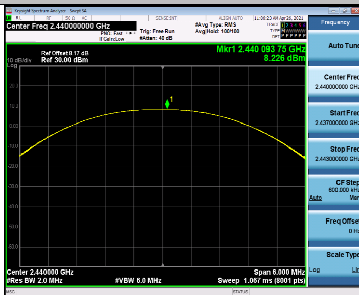
BLE_BT4.2_Ant1_2440
