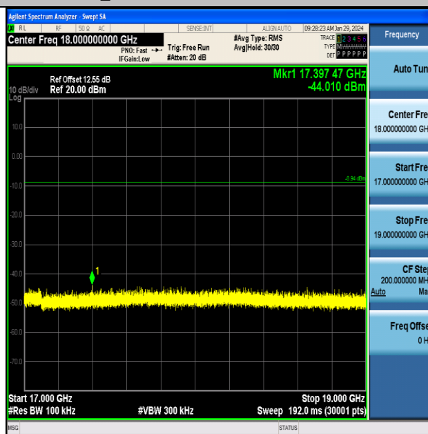
BLE_1M-Ant1-2440-17000~19000-PASS
