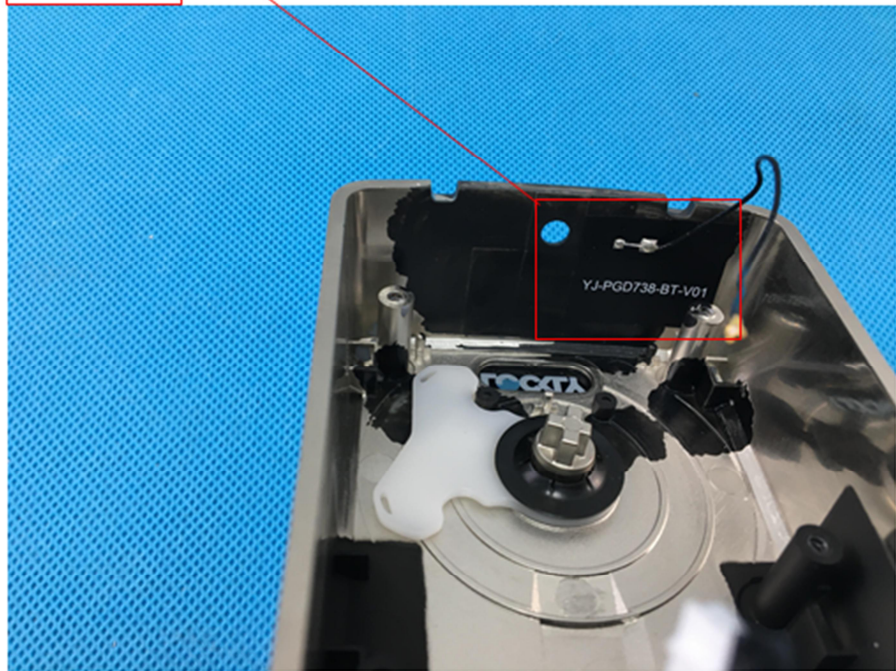
BLE Antenna
