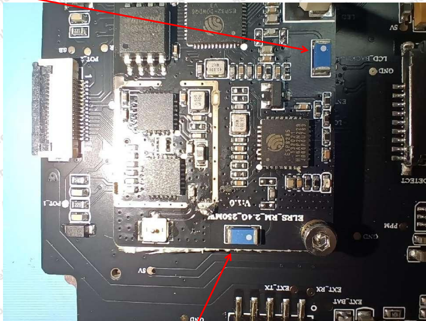
BT ANT
