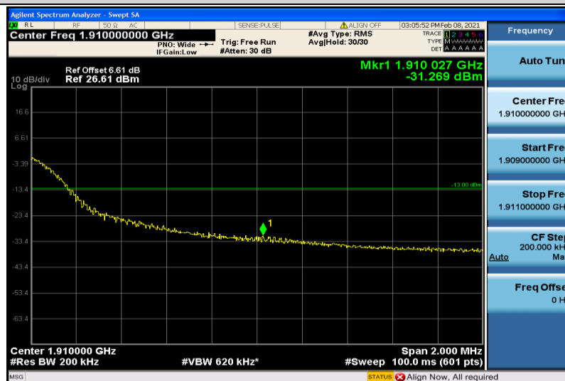
Band2-20MHz-QPSK-19100-6RB#0
