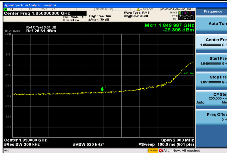
Band2-20MHz-QPSK-18700-6RB#0
