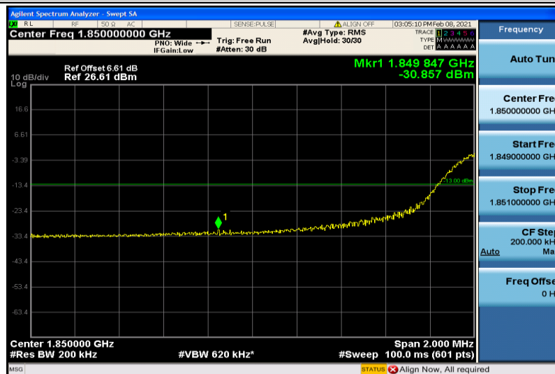
Band2-20MHz-16QAM-18700-6RB#0
