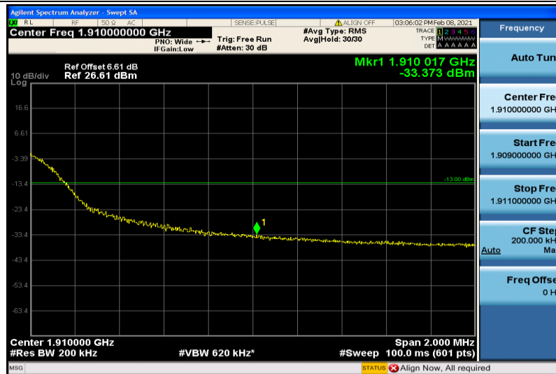
Band2-20MHz-16QAM-19100-6RB#0
