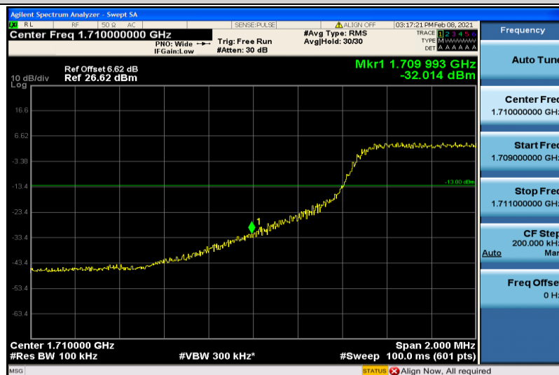
Band4-10MHz-QPSK-20000-6RB#0
