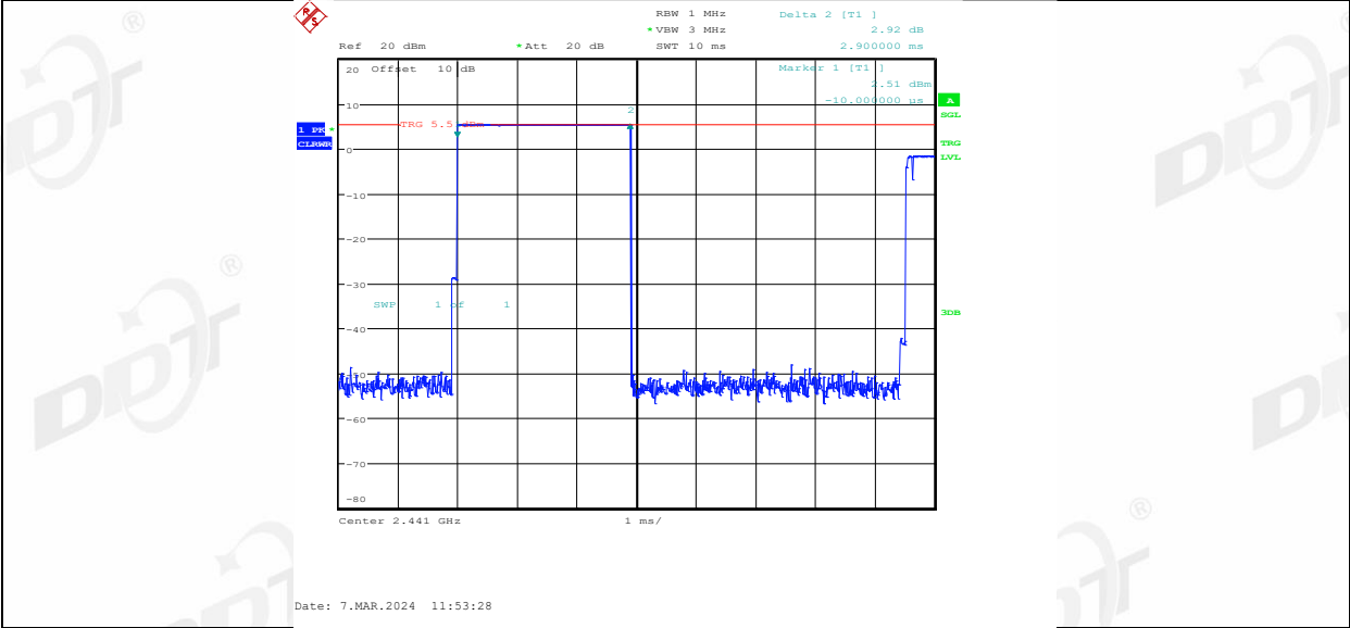
DH5_Ant2_Hop
