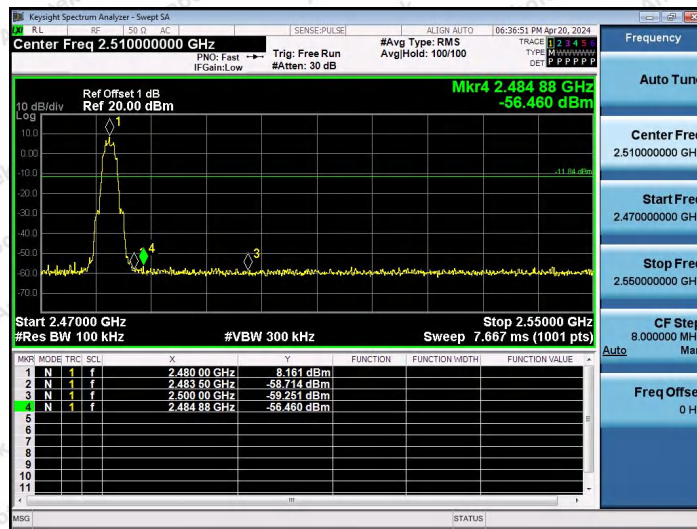
BLE_2M-Ant2-248-PASS
