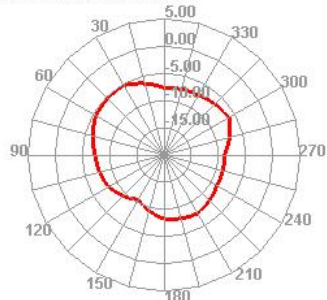
2450.000MHz H
