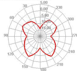
2400.000MHz E2
