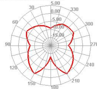
2450.000MHz E2
