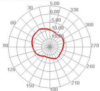
2400.000MHz H
