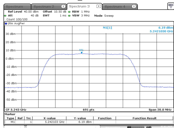
10M_5243MHz
