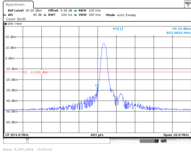
Band26-5MHz-QPSK-26815-1-0-Low--29.10-PASS
