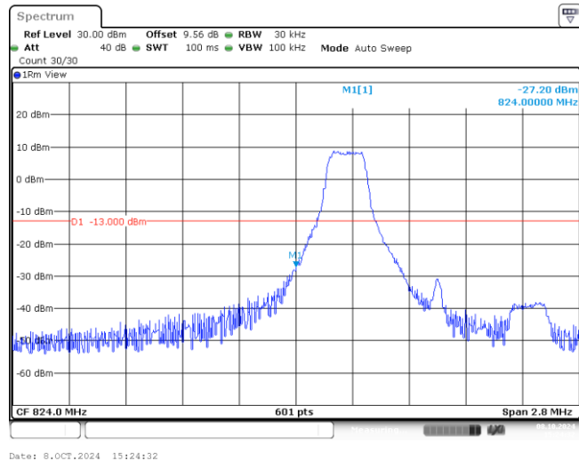
Band26-1.4MHz-QPSK-26797-1-0-Low--27.20-PASS
