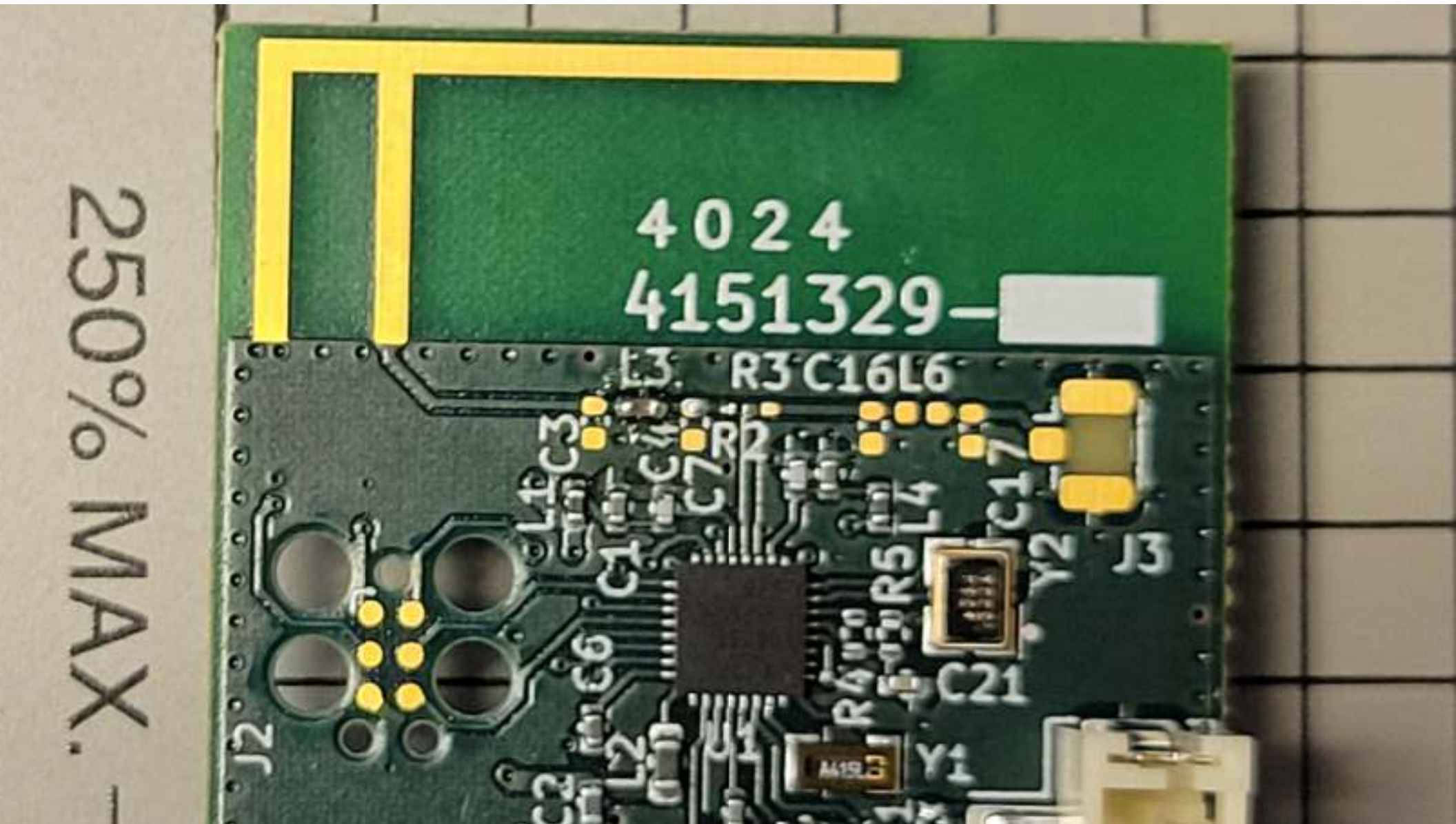
ACTIVE BLE RADIO PCB
