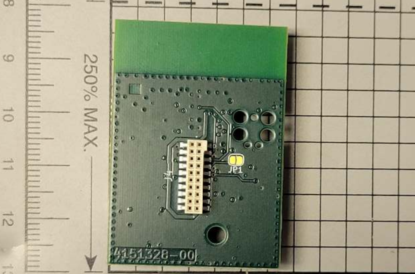
ACTIVE BLE RADIO PCB
