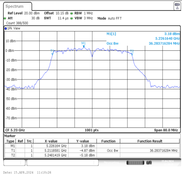
11N40MIMO-Ant2-5230
