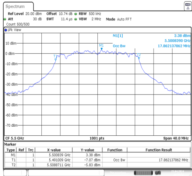
11N20MIMO-Ant2-5500
