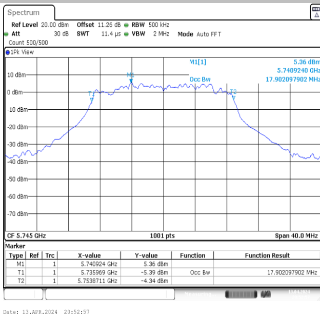
11N20MIMO-Ant1-5745
