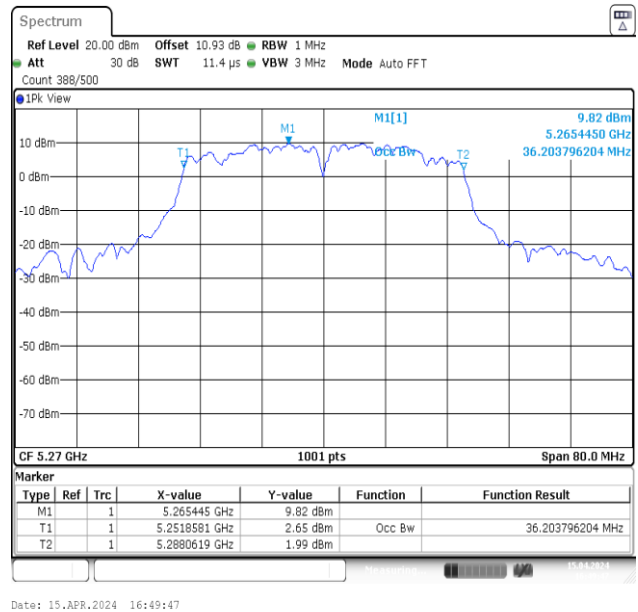
11N40MIMO-Ant2-5270
