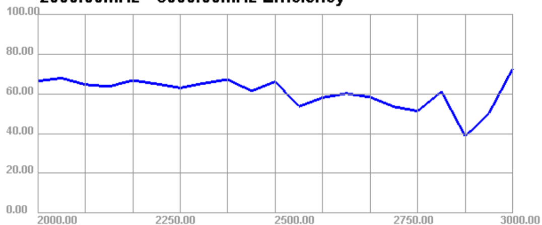
2000.00MHz - 3000.00MHz Efficiency
