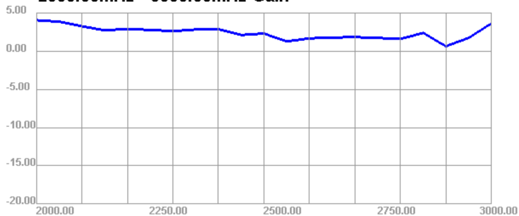
2000.00MHz - 3000.00MHz Gain
