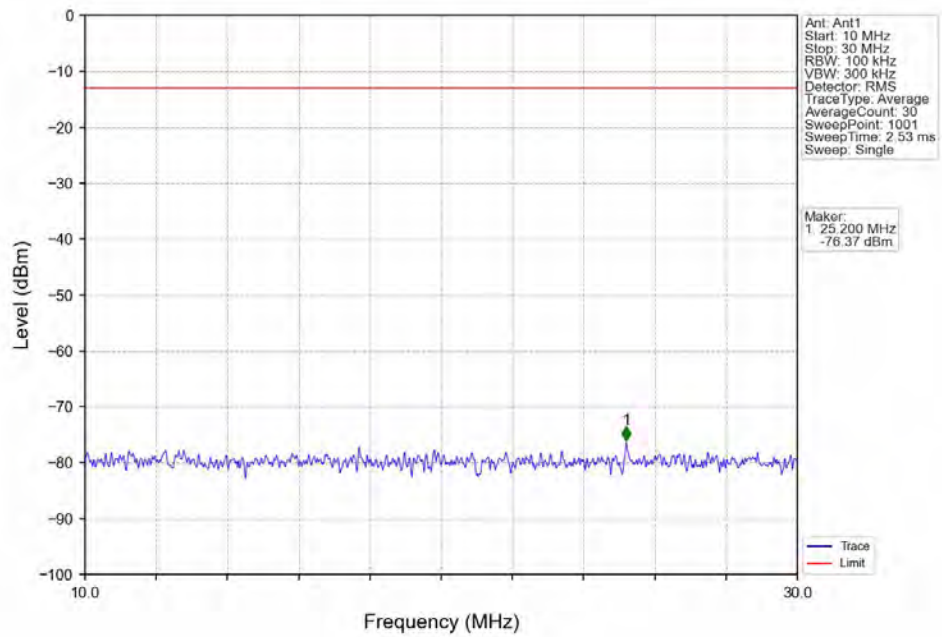
Band12_10MHz_QPSK_MCH_707.5MHz_RB_1_0_NTNV
