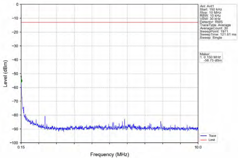
Band12_10MHz_QPSK_MCH_707.5MHz_RB_1_0_NTNV
