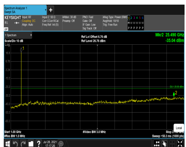
Band41-20MHz-QPSK-40640:1000~27000MHz
