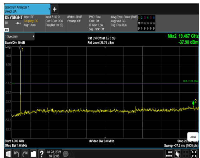
Band25-20MHz-QPSK-26590:1000~20000MHz
