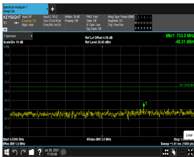
Band41-20MHz-QPSK-40140:30~1000MHz
