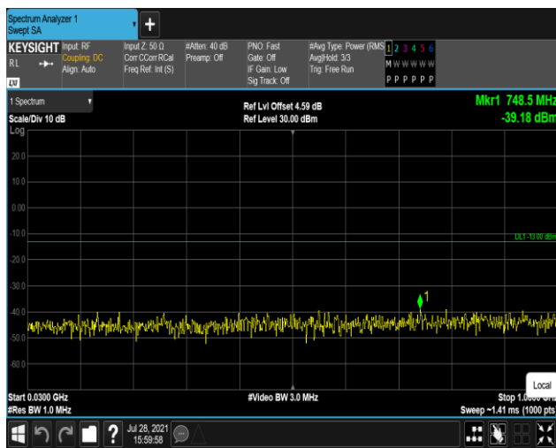
Band25-20MHz-QPSK-26365:30~1000MHz
