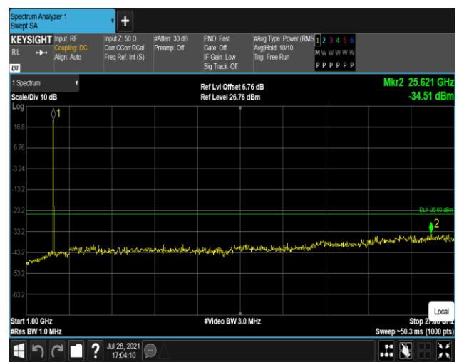
Band41-20MHz-QPSK-40140:1000~27000MHz
