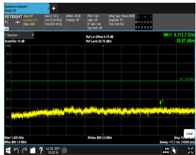
Band26-1.4MHz-QPSK-26783:1000~10000MHz
