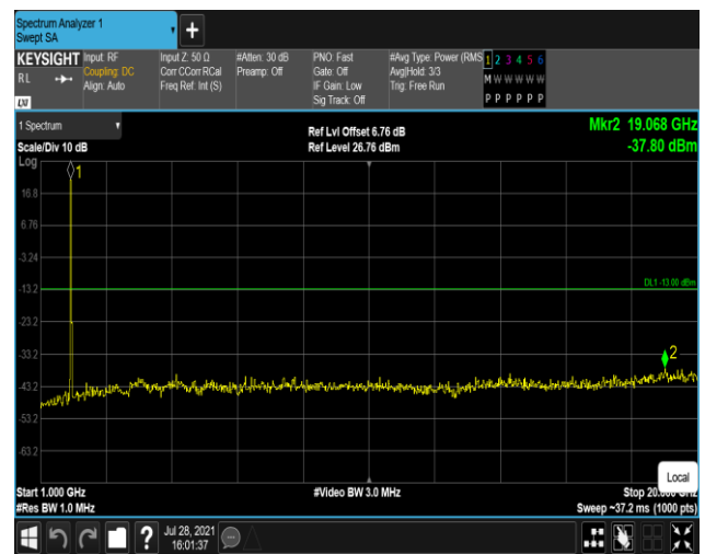
Band25-20MHz-16QAM-26590:1000~20000MHz
