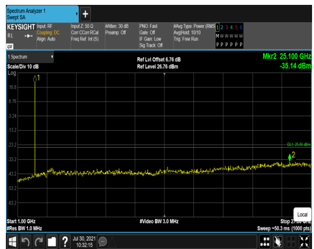
Band41-5MHz-QPSK-40640:1000~27000MHz
