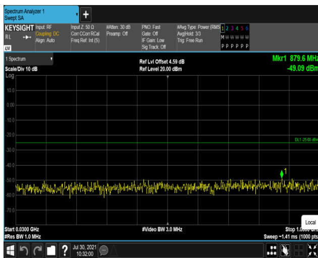
Band41-5MHz-QPSK-40640:30~1000MHz
