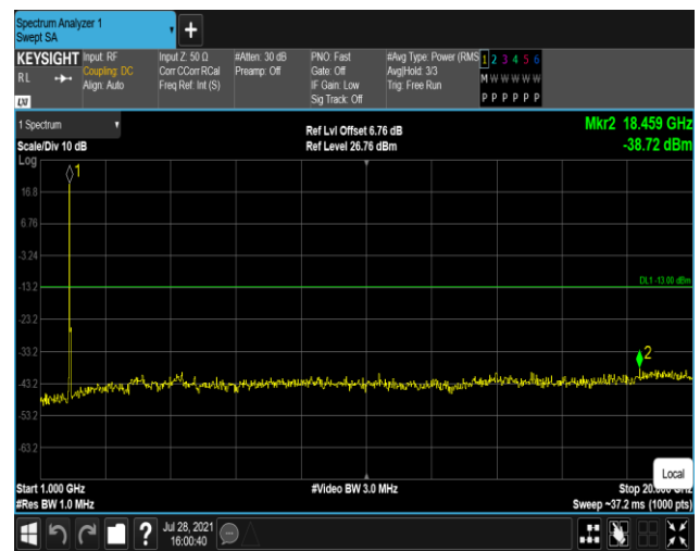
Band25-20MHz-16QAM-26365:1000~20000MHz
