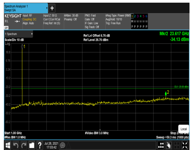
Band41-5MHz-16QAM-40065:1000~27000MHz
