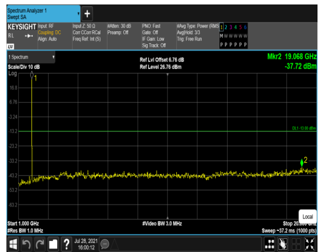
Band25-20MHz-QPSK-26365:1000~20000MHz
