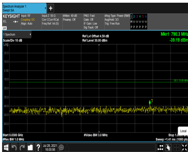
Band25-20MHz-QPSK-26590:30~1000MHz
