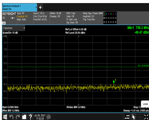
Band41-5MHz-QPSK-40640:30~1000MHz
