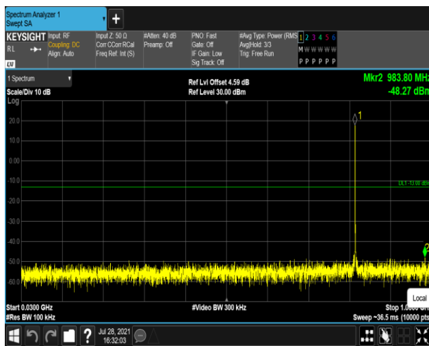
Band26-1.4MHz-QPSK-26783:30~1000MHz
