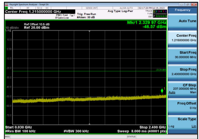
,Plot 3,30MHz~2400MHz-802.11n(HT40) ,2452MHz,Ant2
