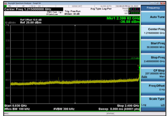
,Plot 3,30MHz~2400MHz-802.11n(HT40) ,2437MHz,Ant2
