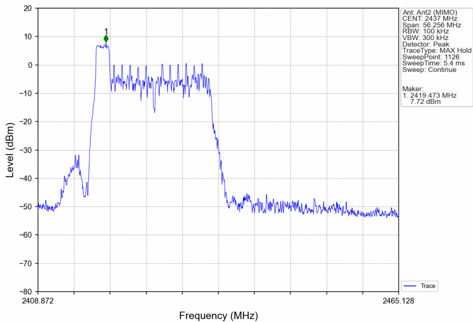
802.11ax(HEW40)_MCH_2437MHz_RU26_Left_Ant2 (MIMO)_NTNV
