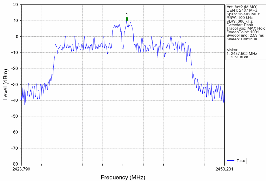
802.11ax(HEW20)_MCH_2437MHz_RU26_Mid_Ant2 (MIMO)_NTNV
