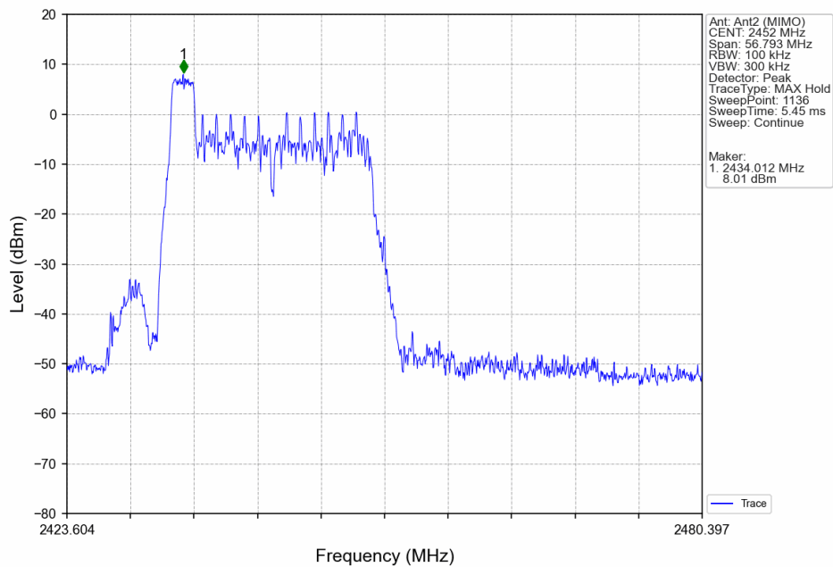
802.11ax(HEW40)_HCH_2452MHz_RU26_Left_Ant2 (MIMO)_NTNV
