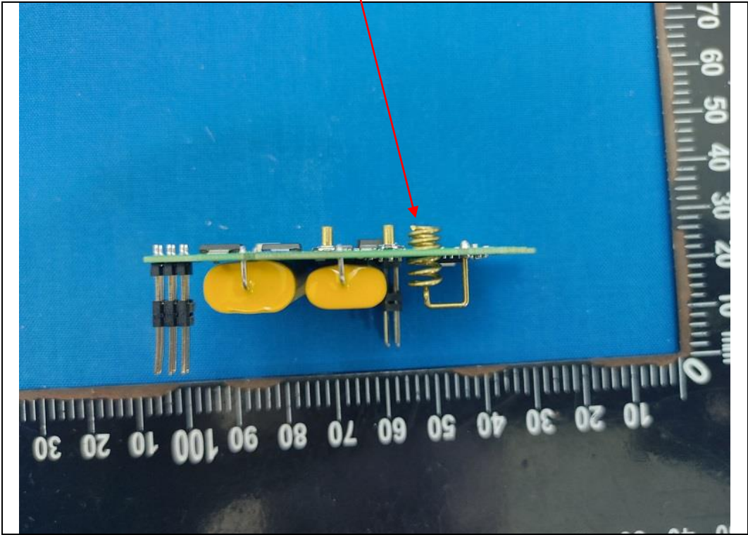
ANTENNA
