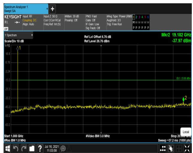
Band4-1.4MHz-QPSK-20393:1000~20000MHz
