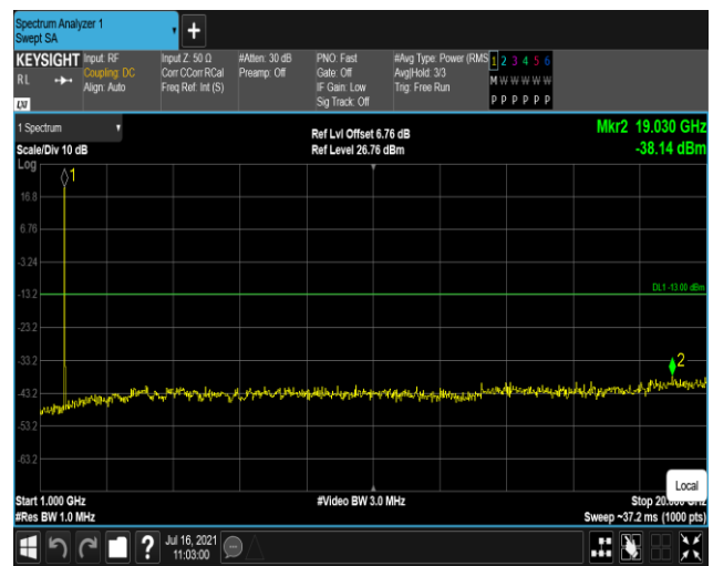
Band4-1.4MHz-QPSK-20175:1000~20000MHz
