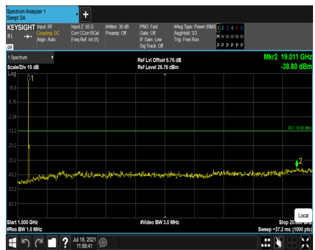
Band4-20MHz-QPSK-20175:1000~20000MHz
