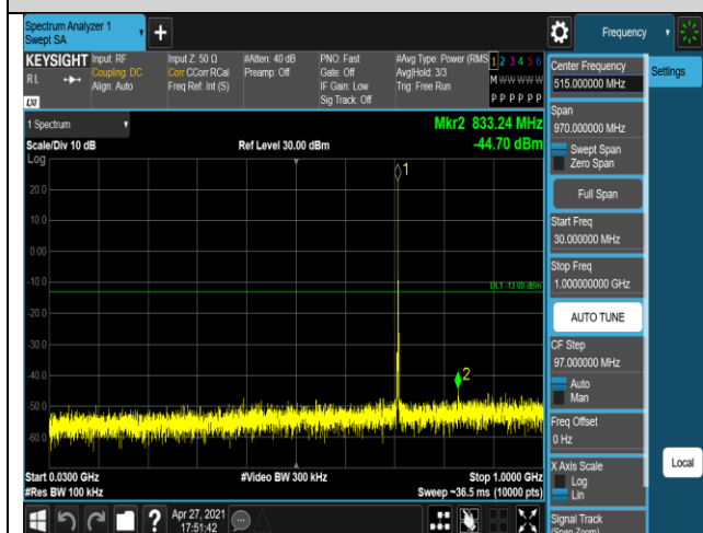
Band12-1.4MHz-16QAM-23017-1RB#0-Range1:30~ 1000MHz
