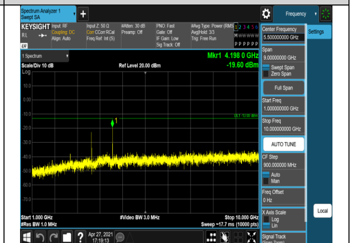
Band12-1.4MHz-QPSK-23017-1RB#0-Range2:1000~1
