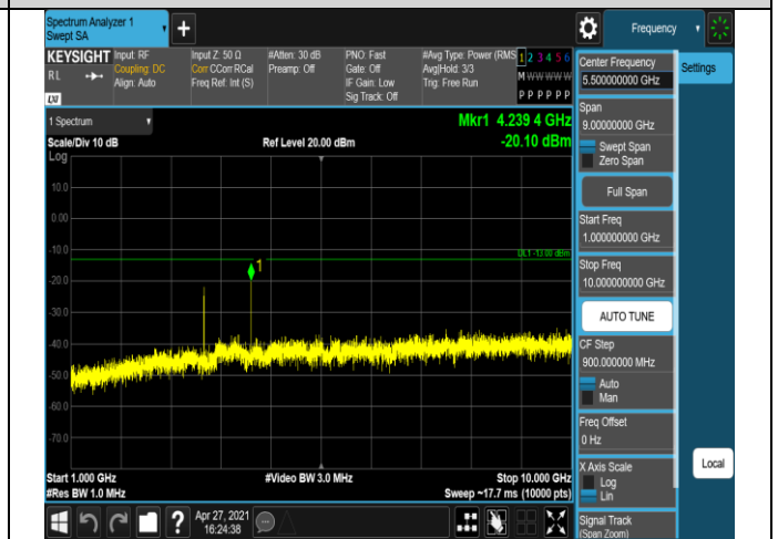
Band5-10MHz-QPSK-20450-1RB#0-Range2:1000~100 00MHz
