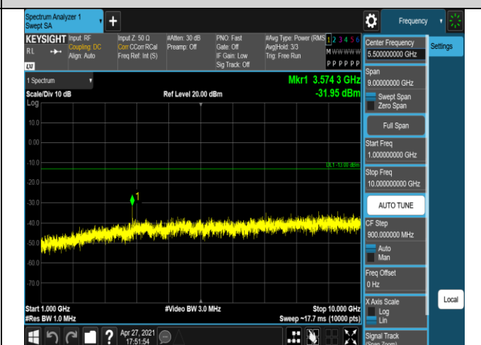
Band12-1.4MHz-16QAM-23017-1RB#0-Range2:1000~ 10000MHz
