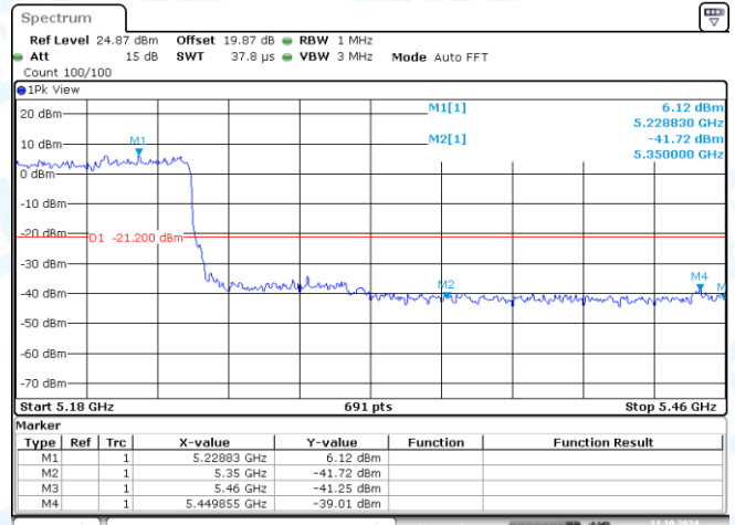
11AX80MIMO-Ant1-5210-PASS
