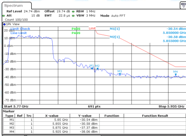
11AX40MIMO-Ant1-5755-PASS
