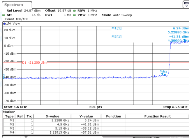
11AX80MIMO-Ant1-5210-PASS
