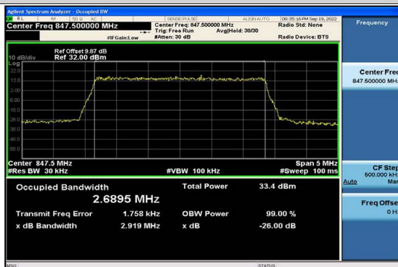
Band5-3MHz-QPSK-20635-15RB#0-2.6895
