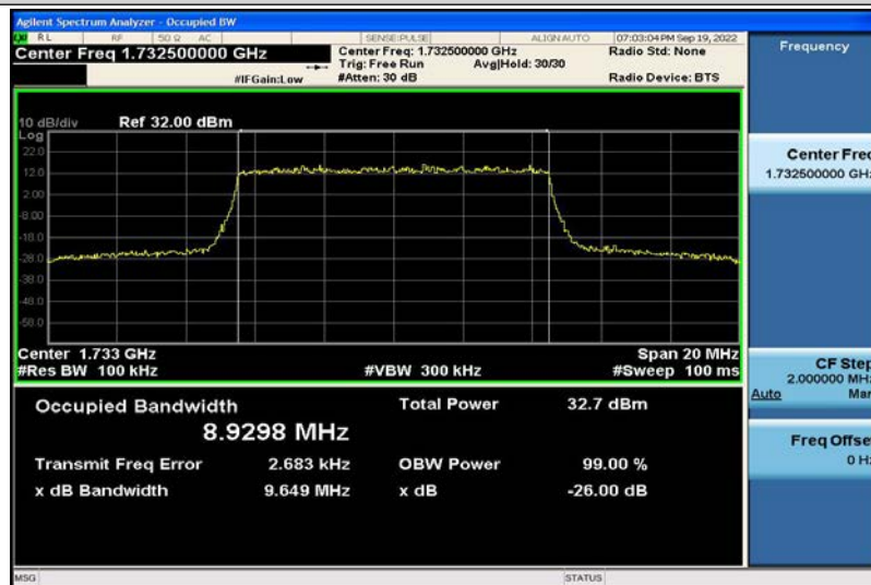
Band4-10MHz-QPSK-20175-50RB#0-8.9298
