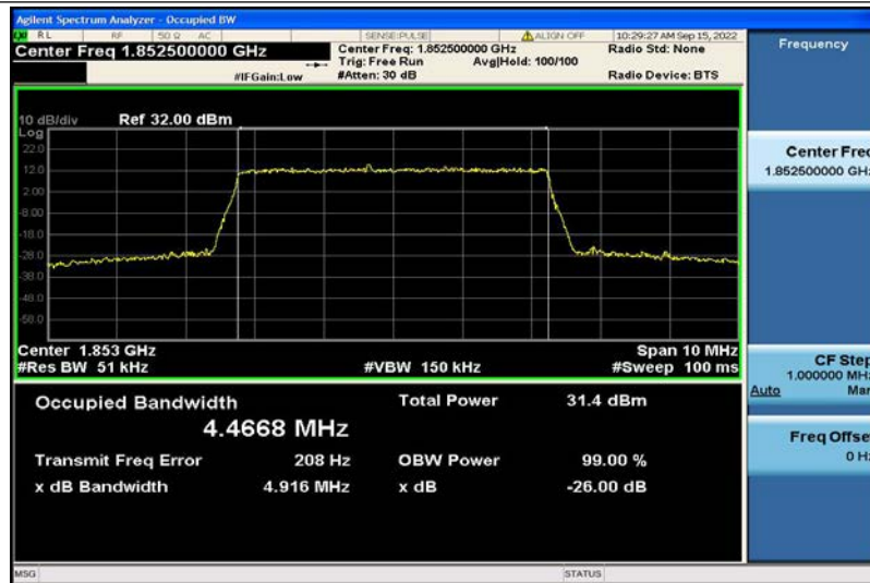
Band2-5MHz-QPSK-18625-25RB#0-4.4668
