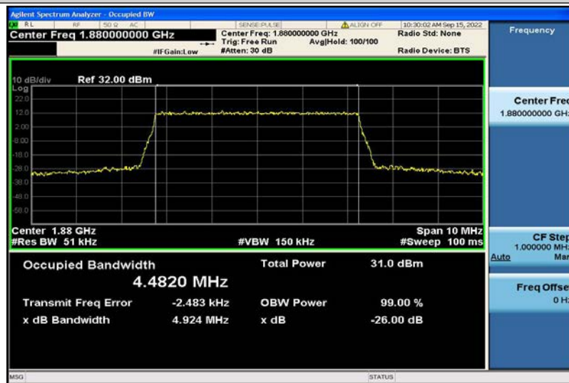
Band2-5MHz-QPSK-18900-25RB#0-4.4820
