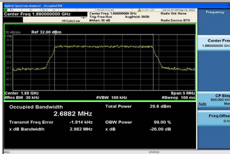
Band2-3MHz-QPSK-18900-15RB#0-2.6882
