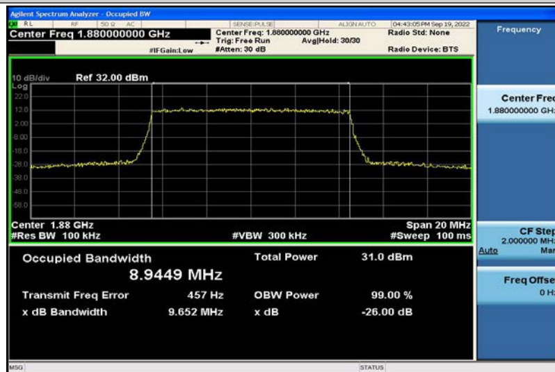
Band2-10MHz-16QAM-18900-50RB#0-8.9449
