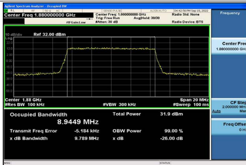
Band2-10MHz-QPSK-18900-50RB#0-8.9449
