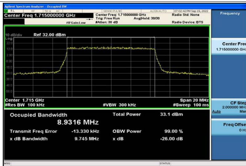
Band4-10MHz-QPSK-20000-50RB#0-8.9316
