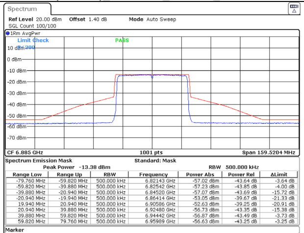
802.11ax (40MHz) 6885MHz Chain B NSS-1
