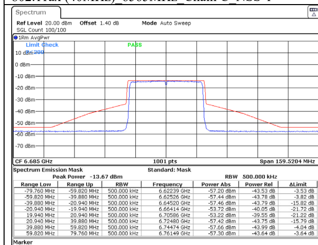
802.11ax (40MHz) 6685MHz Chain A NSS-1
