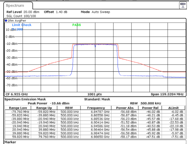
802.11ax (40MHz) 6925MHz Chain D NSS-1
