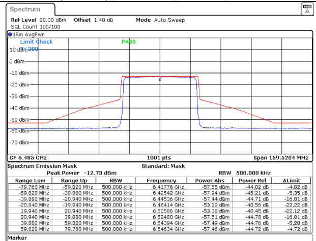
802.11ax (40MHz) 6485MHz Chain D NSS-1
