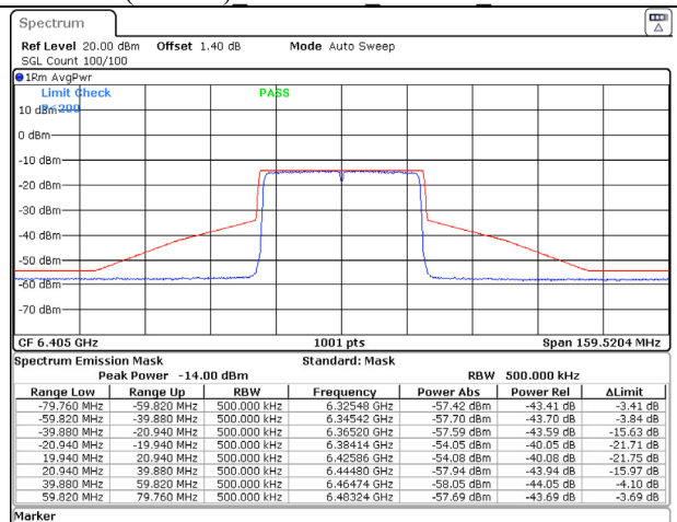
802.11ax (40MHz) 6405MHz Chain D NSS-1
