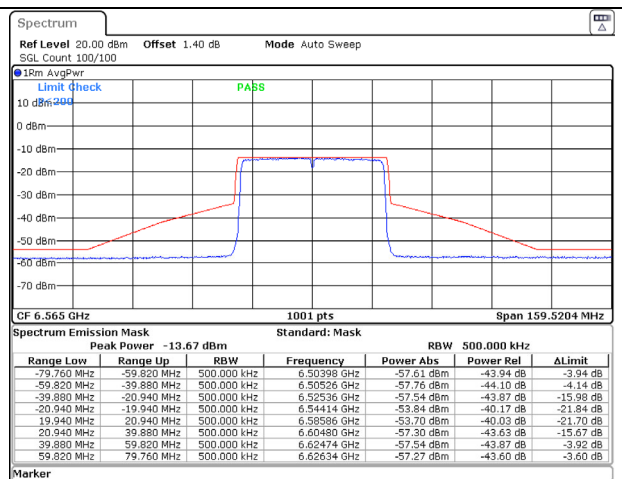
802.11ax (40MHz) 6565MHz Chain D NSS-1
