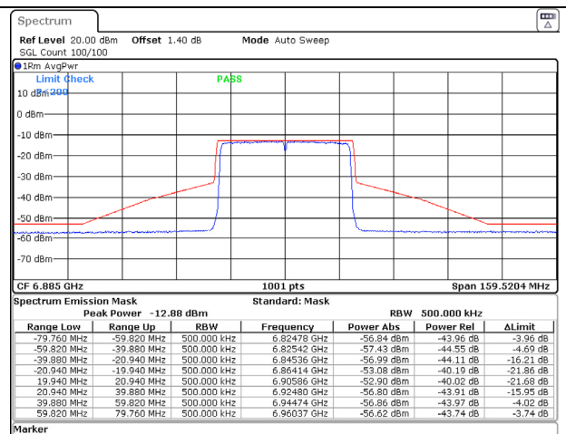
802.11ax (40MHz) 6885MHz Chain D NSS-1
