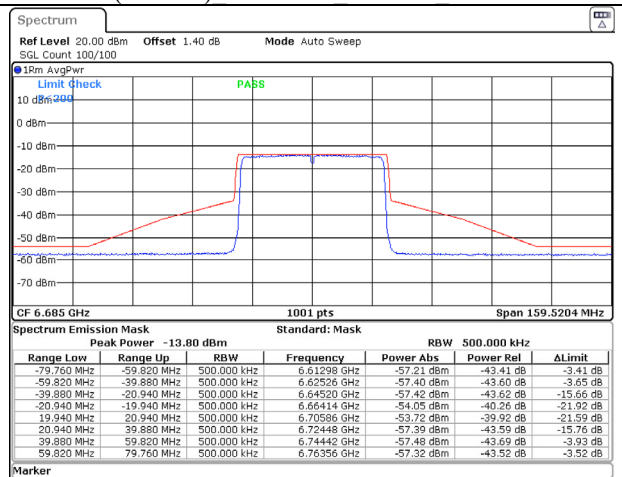
802.11ax (40MHz) 6685MHz Chain D NSS-1
