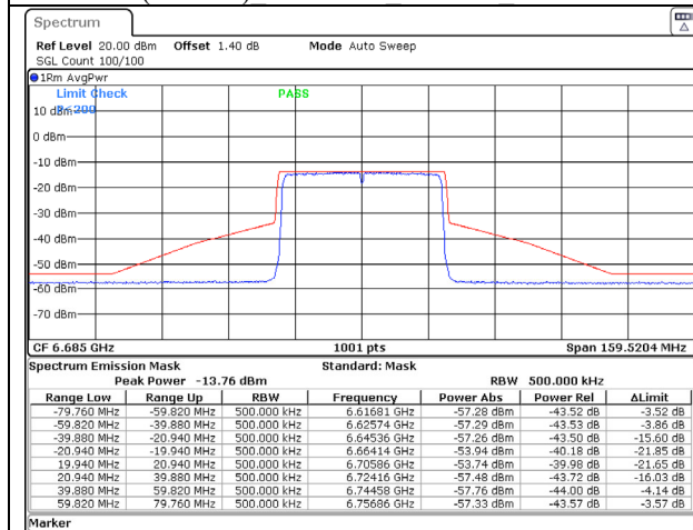
802.11ax (40MHz) 6685MHz Chain C NSS-1
