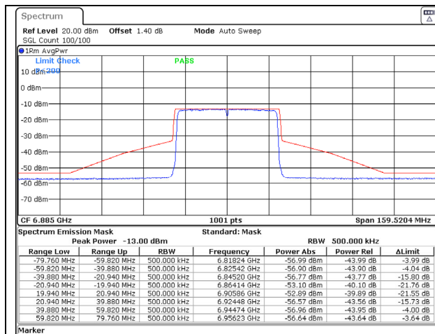
802.11ax (40MHz) 6885MHz Chain C NSS-1
