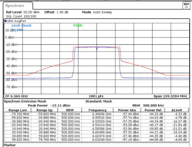
802.11ax (40MHz) 6565MHz Chain B NSS-1
