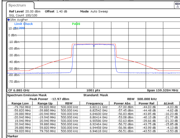
802.11ax (40MHz) 6885MHz Chain A NSS-1
