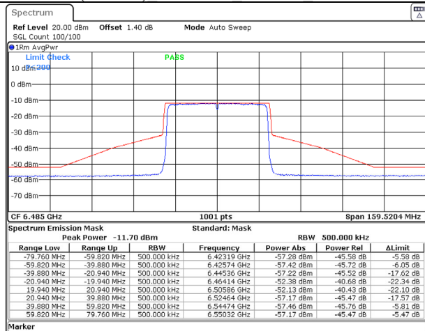
802.11ax (40MHz) 6485MHz Chain C NSS-1
