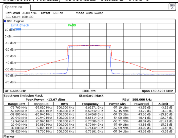
802.11ax (40MHz) 6685MHz Chain B NSS-1
