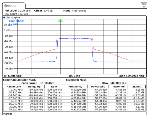
802.11ax (40MHz) 6405MHz Chain B NSS-1
