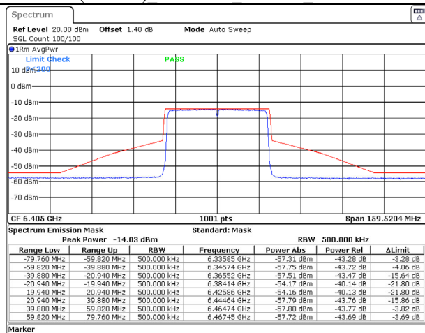
802.11ax (40MHz) 6405MHz Chain A NSS-1
