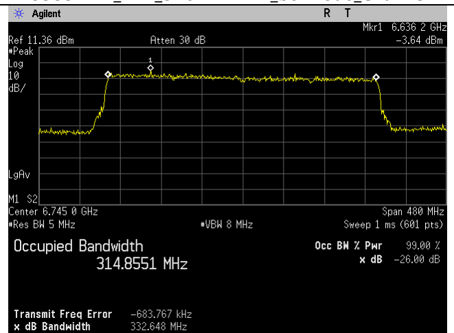
6745MHz_159_320MHz BW_be-mode_Chain 1
