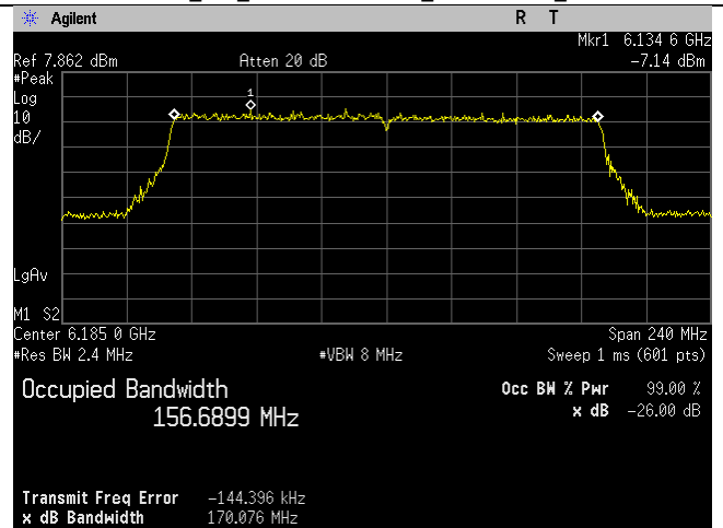
6185MHz_47_160MHz BW_be-mode_Chain 1
