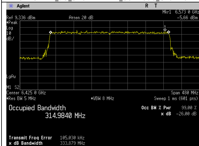
6425MHz_95_320MHz BW_be-mode_Chain 2
