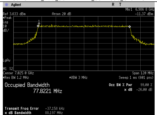
7025MHz_215_80MHz BW_be-mode_Chain 1
