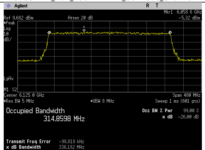
6125MHz_31_320MHz BW_be-mode_Chain 1
