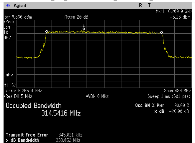
6265MHz_63_320MHz BW_be-mode_Chain 3
