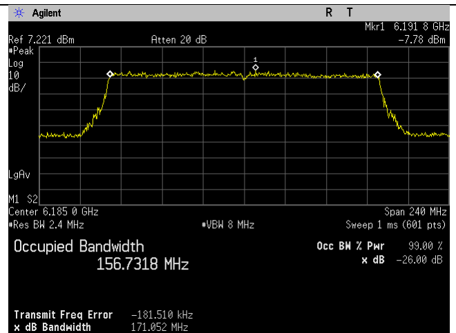
6185MHz_47_160MHz BW_be-mode_Chain 3
