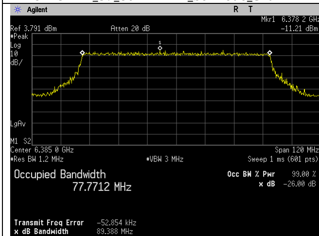
6385MHz_87_80MHz BW_be-mode_Chain 0
