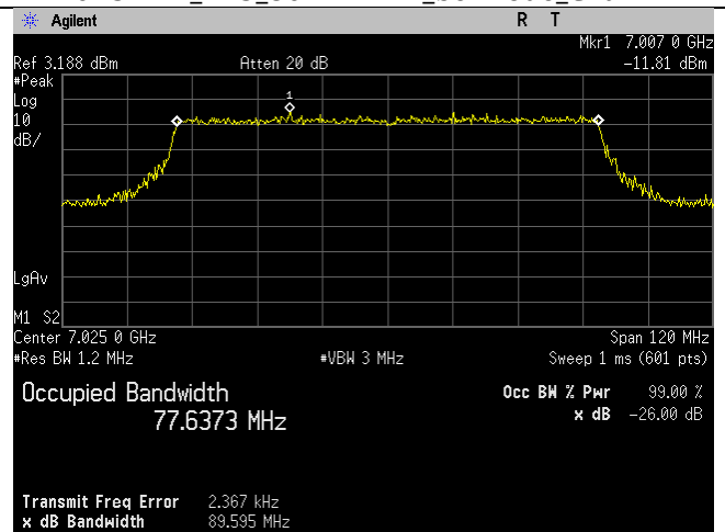
7025MHz_215_80MHz BW_be-mode_Chain 3
