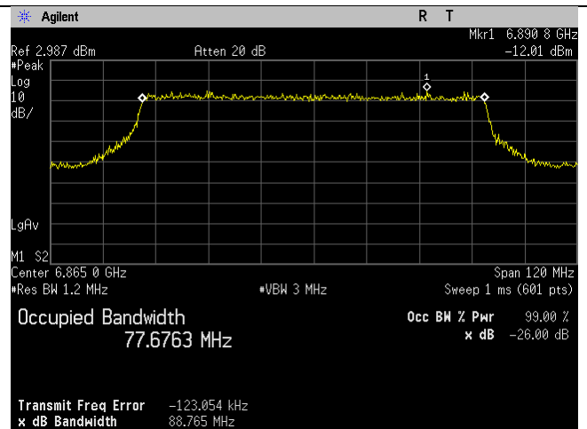
6865MHz_183_80MHz BW_be-mode_Chain 1
