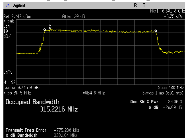
6745MHz_159_320MHz BW_be-mode_Chain 3
