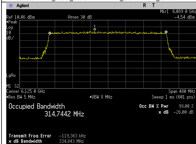
6125MHz_31_320MHz BW_be-mode_Chain 0
