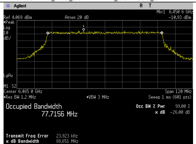
6465MHz_103_80MHz BW_be-mode_Chain 3
