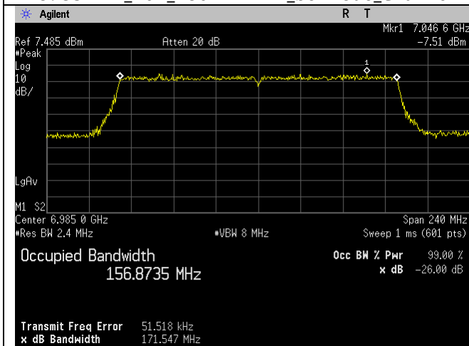
6985MHz_207_160MHz BW_be-mode_Chain 2
