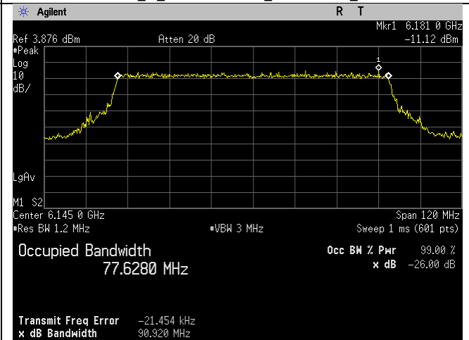
6145MHz_39_80MHz BW_be-mode_Chain 1
