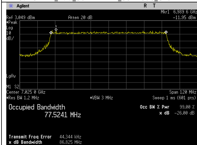
7025MHz_215_80MHz BW_be-mode_Chain 0
