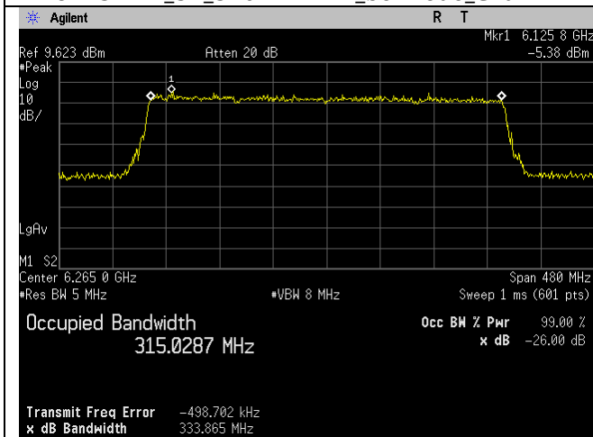
6265MHz_63_320MHz BW_be-mode_Chain 0
