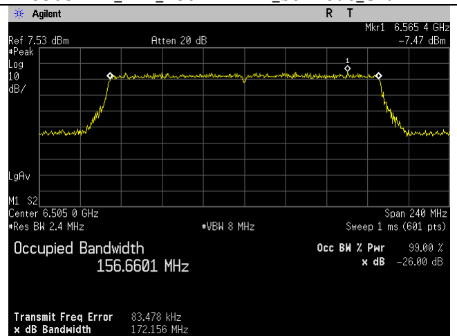
6505MHz_111_160MHz BW_be-mode_Chain 3
