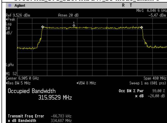
6905MHz_191_320MHz BW_be-mode_Chain 2
