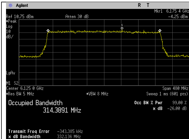
6125MHz_31_320MHz BW_be-mode_Chain 2
