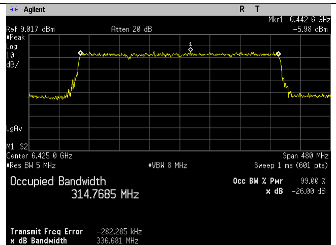
6425MHz_95_320MHz BW_be-mode_Chain 1
