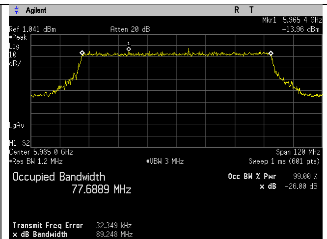
5985MHz_7_80MHz BW_be-mode_Chain 1
