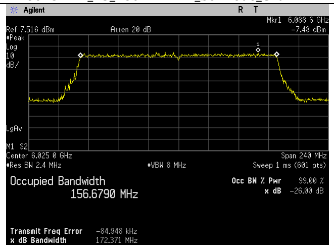
6025MHz_15_160MHz BW_be-mode_Chain 3
