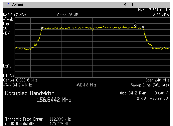
6985MHz_207_160MHz BW_be-mode_Chain 1
