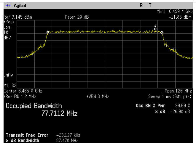
6465MHz_103_80MHz BW_be-mode_Chain 1
