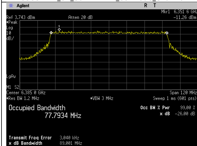
6385MHz_87_80MHz BW_be-mode_Chain 2
