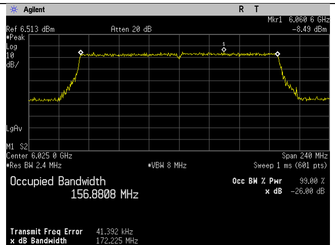
6025MHz_15_160MHz BW_be-mode_Chain 1
