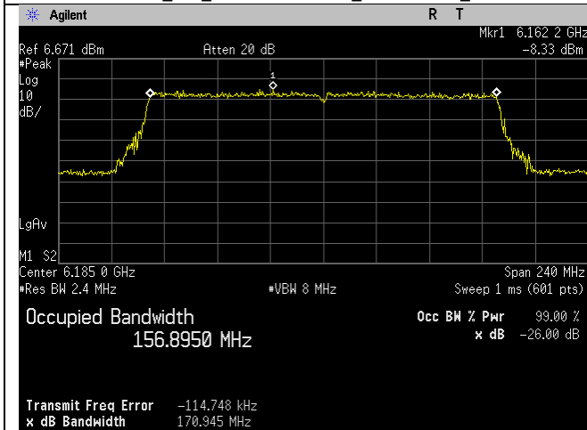
6185MHz_47_160MHz BW_be-mode_Chain 0
