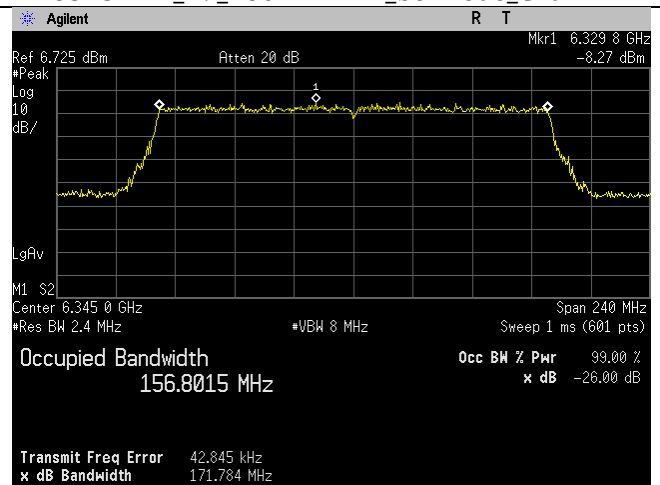
6345MHz_79_160MHz BW_be-mode_Chain 3
