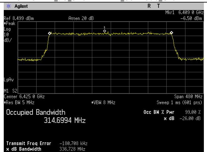
6425MHz_95_320MHz BW_be-mode_Chain 3
