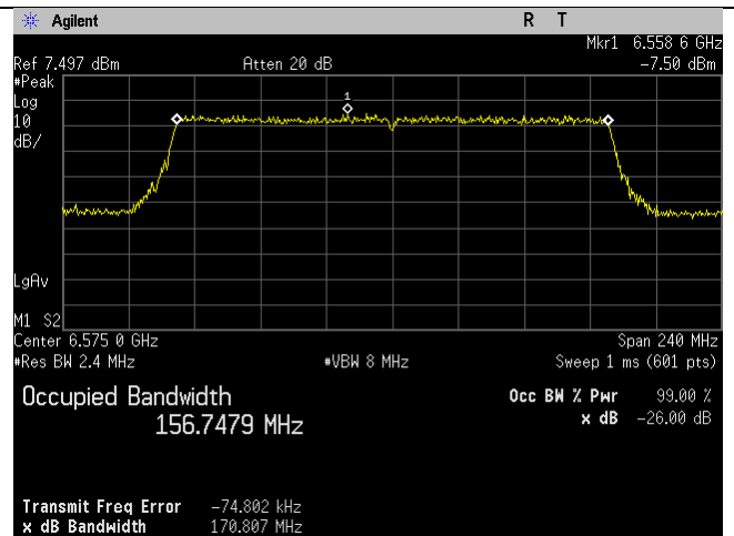
6575MHz_143_160MHz BW_be-mode_Chain 3
