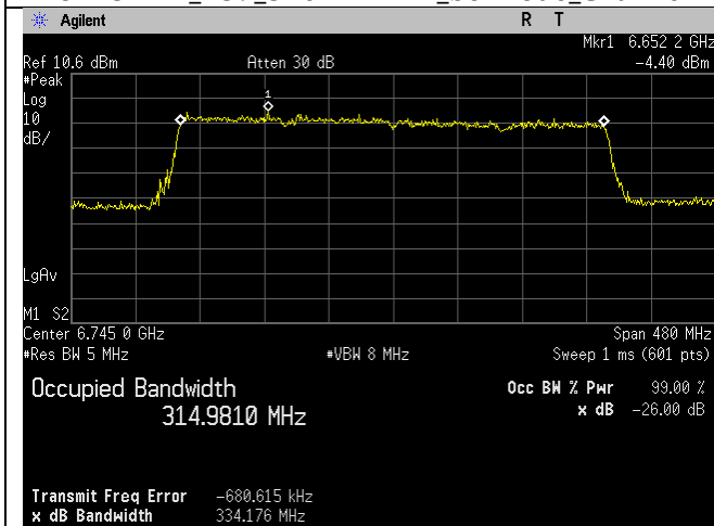
6745MHz_159_320MHz BW_be-mode_Chain 2
