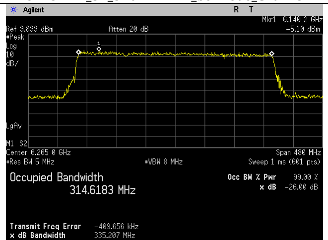
6265MHz_63_320MHz BW_be-mode_Chain 1
