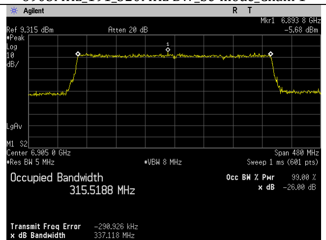
6905MHz_191_320MHz BW_be-mode_Chain 3
