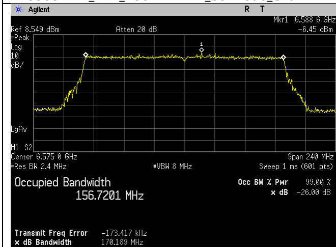
6575MHz_143_160MHz BW_be-mode_Chain 0
