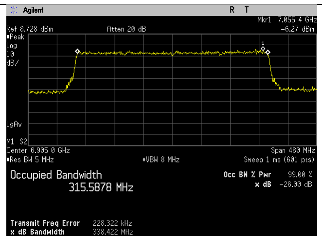
6905MHz_191_320MHz BW_be-mode_Chain 1
