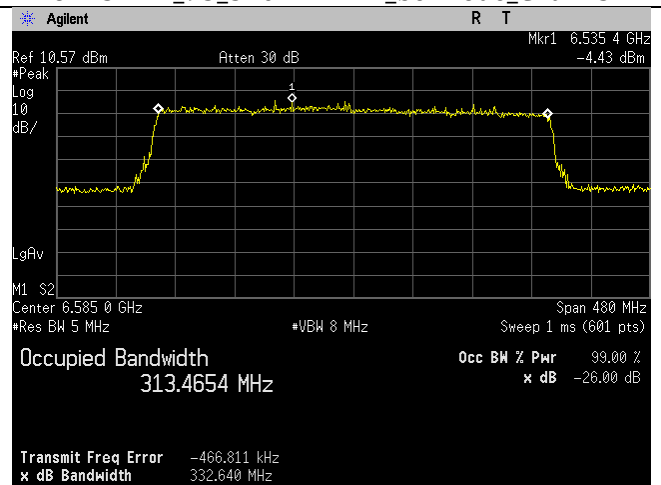
6585MHz_127_320MHz BW_be-mode_Chain 1
