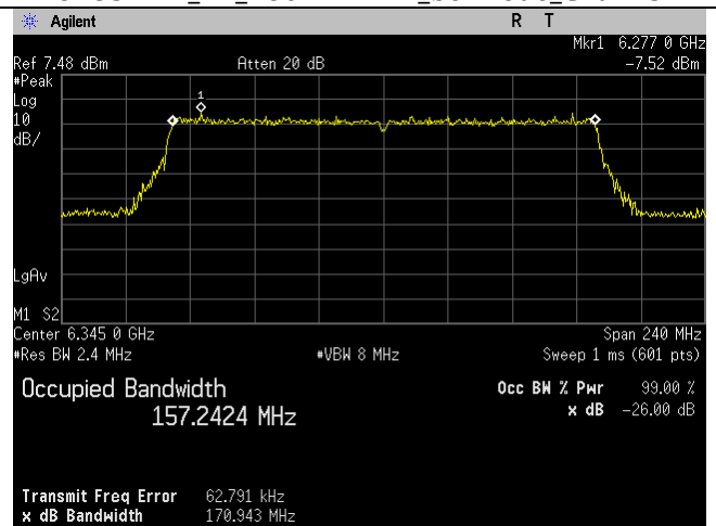
6345MHz_79_160MHz BW_be-mode_Chain 1
