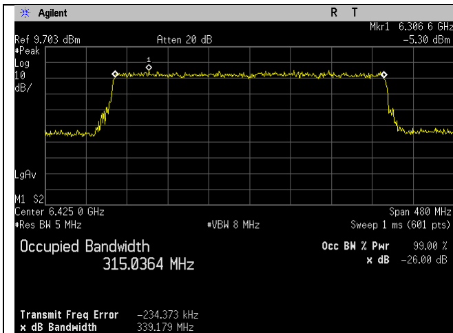
6425MHz_95_320MHz BW_be-mode_Chain 0
