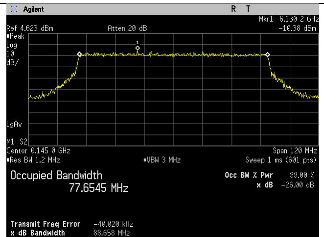
6145MHz_39_80MHz BW_be-mode_Chain 3
