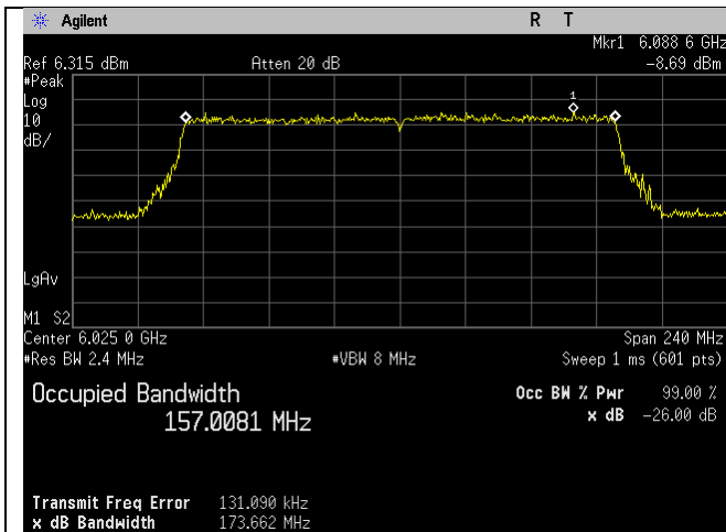
6025MHz_15_160MHz BW_be-mode_Chain 0
