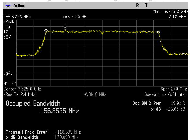
6825MHz_175_160MHz BW_be-mode_Chain 1
