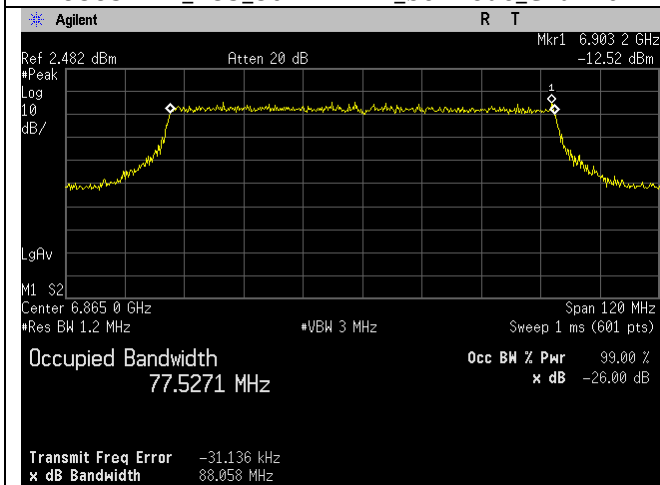
6865MHz_183_80MHz BW_be-mode_Chain 2
