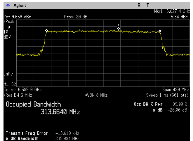
6585MHz_127_320MHz BW_be-mode_Chain 3
