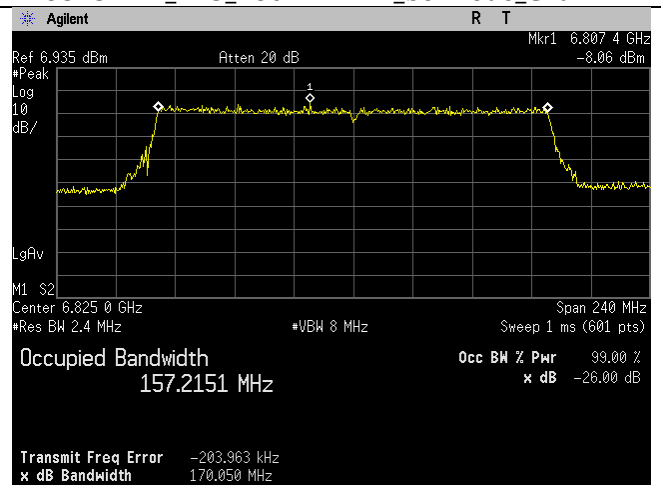
6825MHz_175_160MHz BW_be-mode_Chain 3
