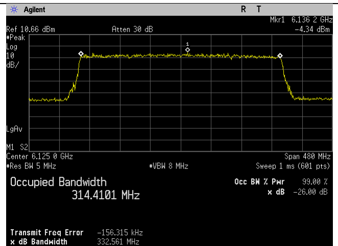
6125MHz_31_320MHz BW_be-mode_Chain 3
