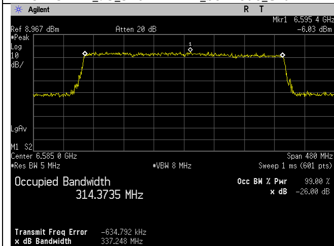
6585MHz_127_320MHz BW_be-mode_Chain 0
