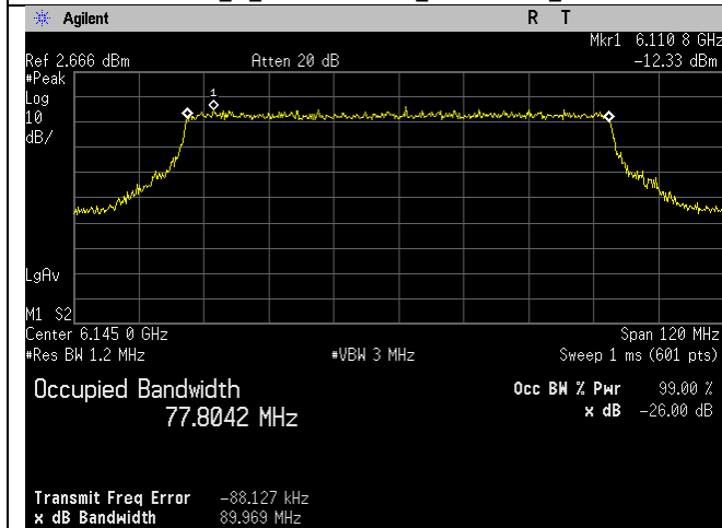
6145MHz_39_80MHz BW_be-mode_Chain 0
