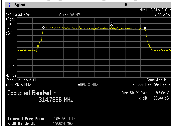
6265MHz_63_320MHz BW_be-mode_Chain 2
