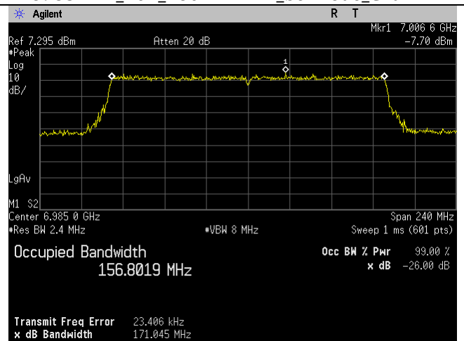
6985MHz_207_160MHz BW_be-mode_Chain 3
