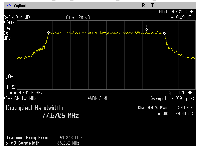
6705MHz_151_80MHz BW_be-mode_Chain 3
