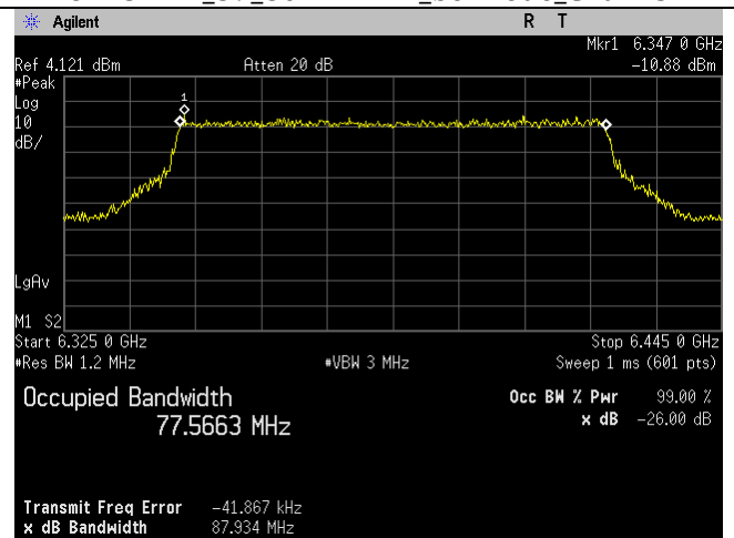
6385MHz_87_80MHz BW_be-mode_Chain 1
