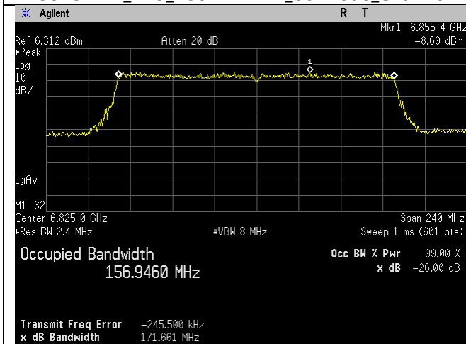
6825MHz_175_160MHz BW_be-mode_Chain 2
