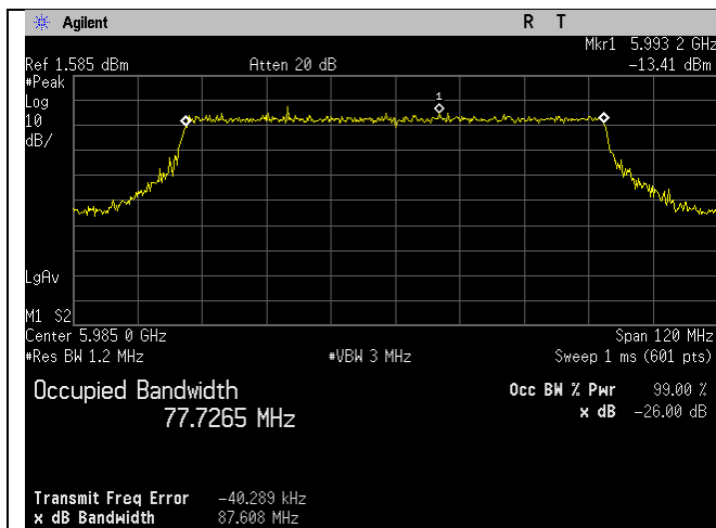
5985MHz_7_80MHz BW_be-mode_Chain 0
