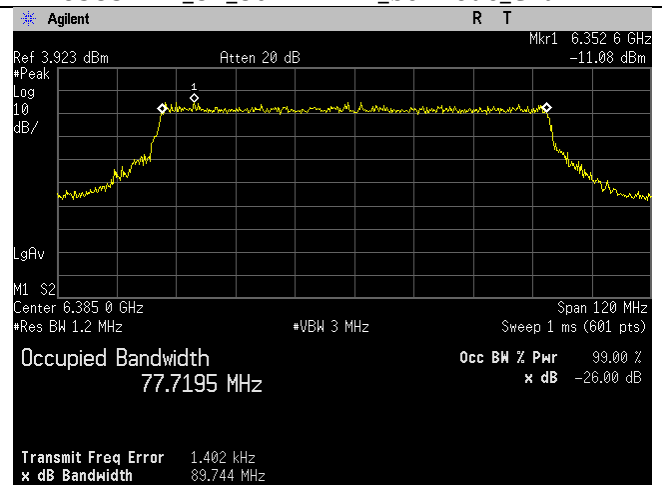
6385MHz_87_80MHz BW_be-mode_Chain 3
