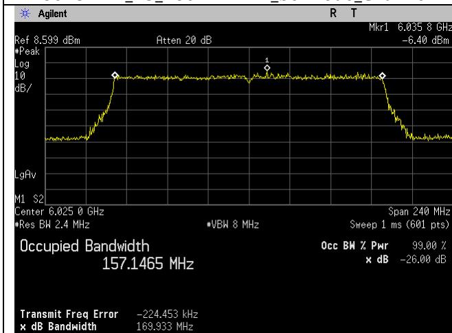
6025MHz_15_160MHz BW_be-mode_Chain 2
