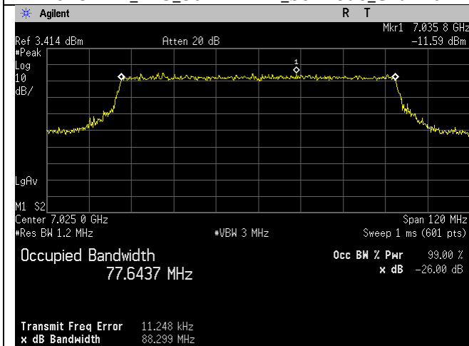
7025MHz_215_80MHz BW_be-mode_Chain 2
