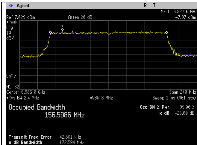
6985MHz_207_160MHz BW_be-mode_Chain 0
