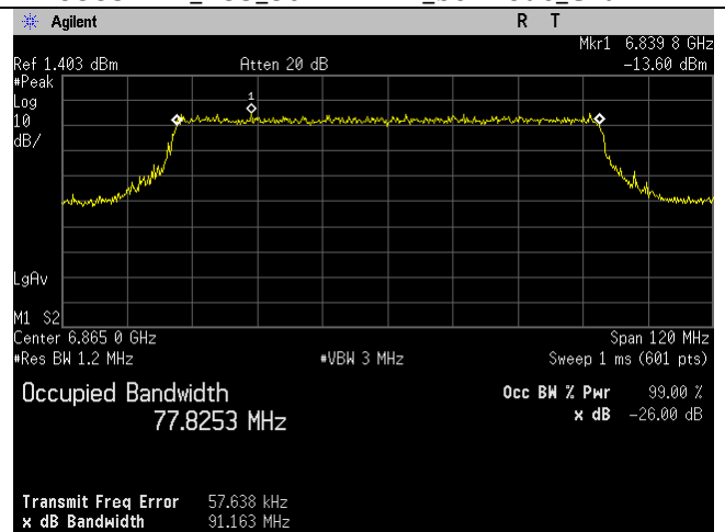
6865MHz_183_80MHz BW_be-mode_Chain 3
