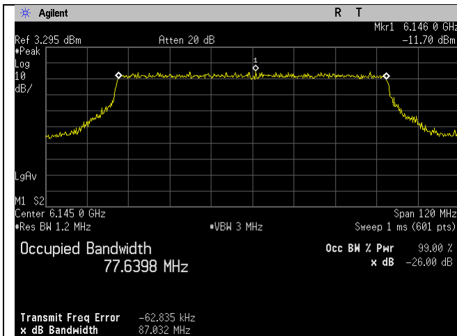
6145MHz_39_80MHz BW_be-mode_Chain 2
