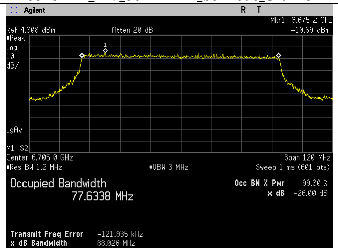
6705MHz_151_80MHz BW_be-mode_Chain 1
