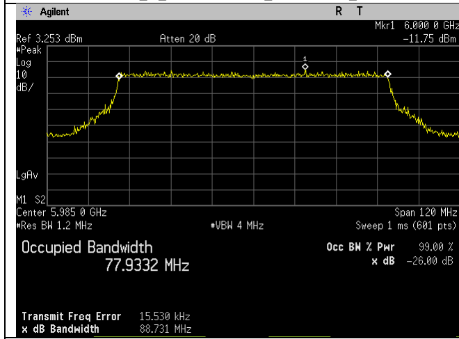
5985MHz_7_80MHz BW_be-mode_Chain 2
