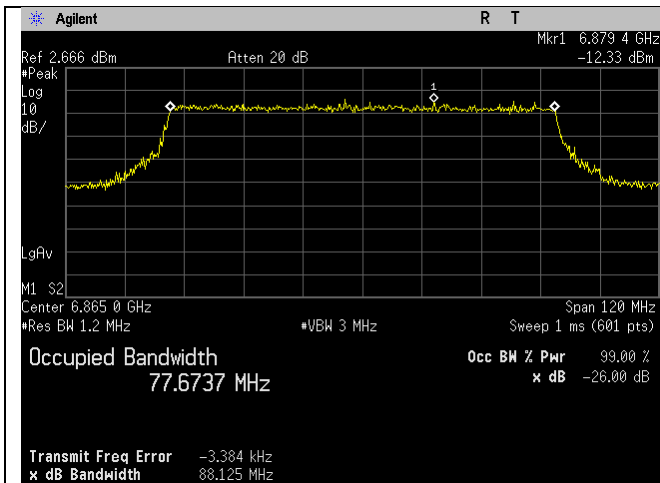
6865MHz_183_80MHz BW_be-mode_Chain 0
