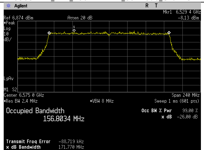
6575MHz_143_160MHz BW_be-mode_Chain 1
