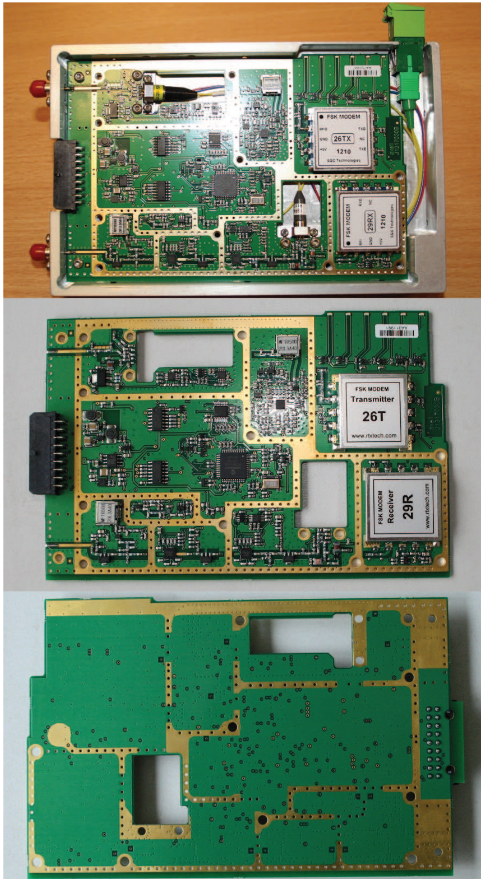
J1311001 FO module
