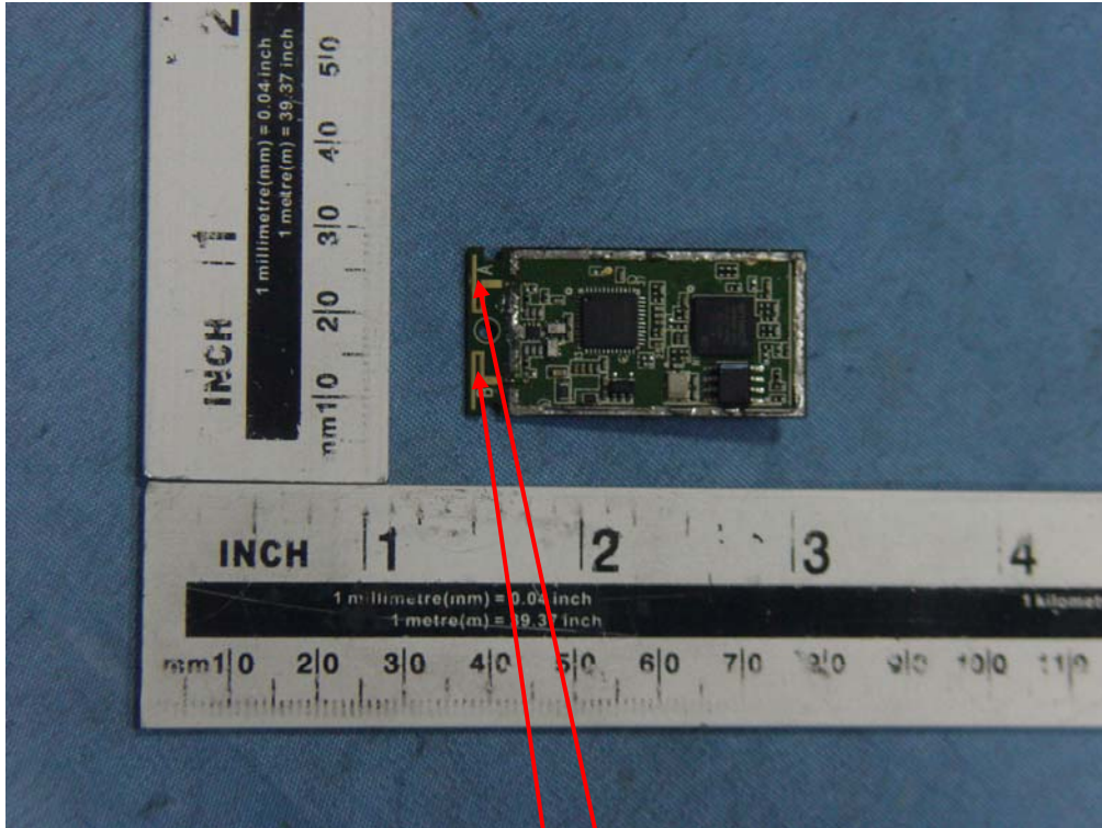
5.8GHz Antenna
