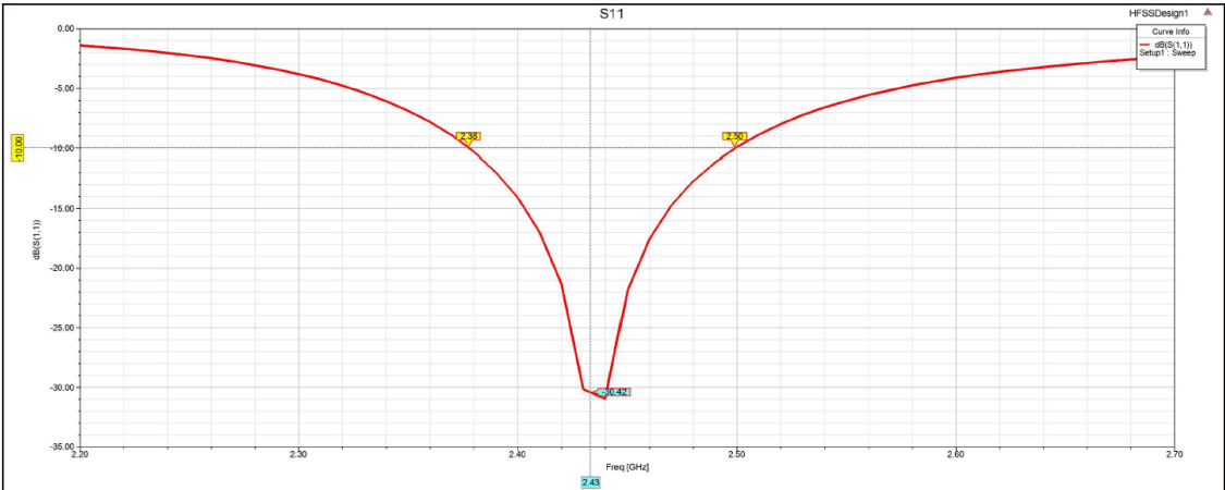
天线S11
