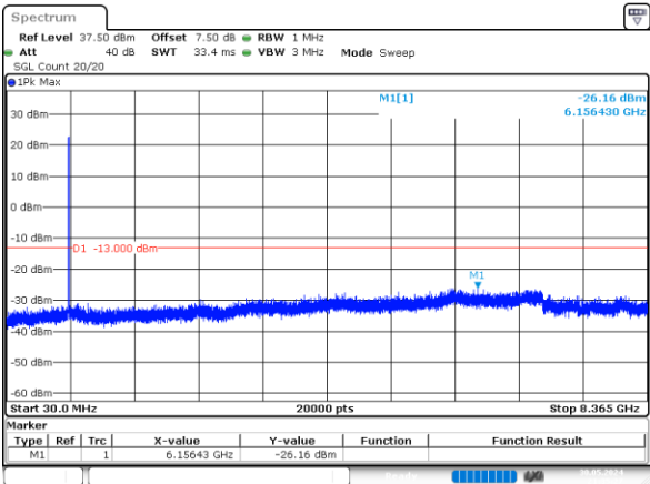
3MHz_Middle_QPSK_15@0 -26.16dBm
