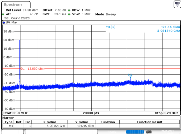
10MHz_Low_QPSK_50@0 -24.45dBm
