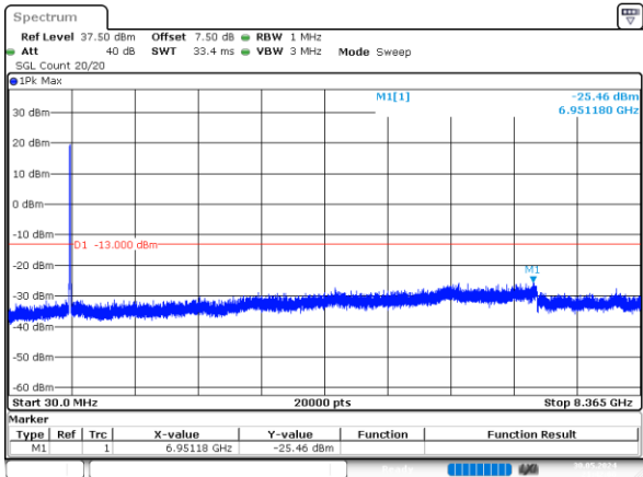
10MHz_Middle_QPSK_50@0 -25.46dBm
