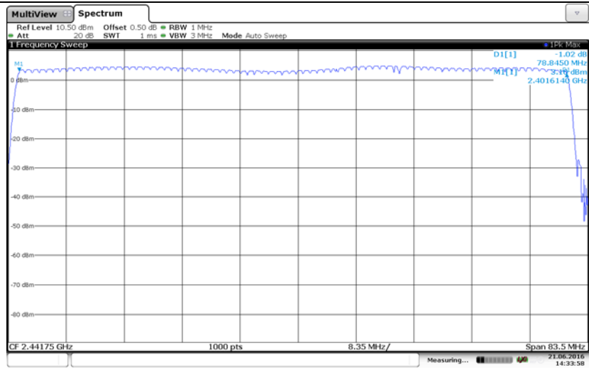
GFSK
