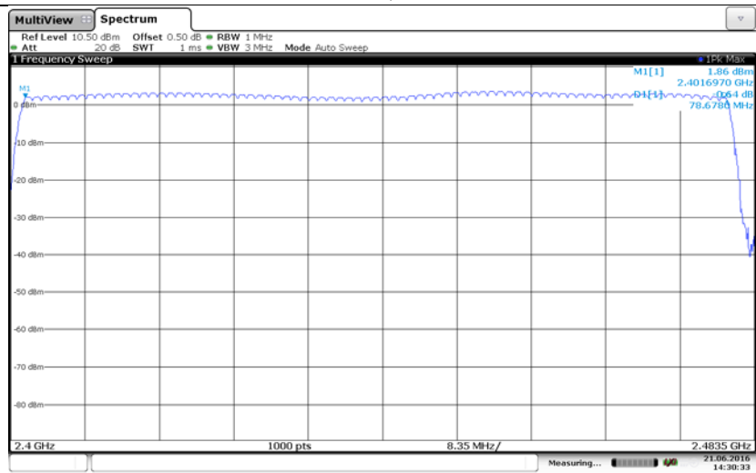
8DPSK
