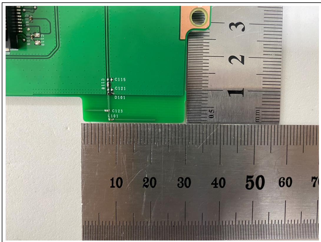
<WLAN Antenna>
