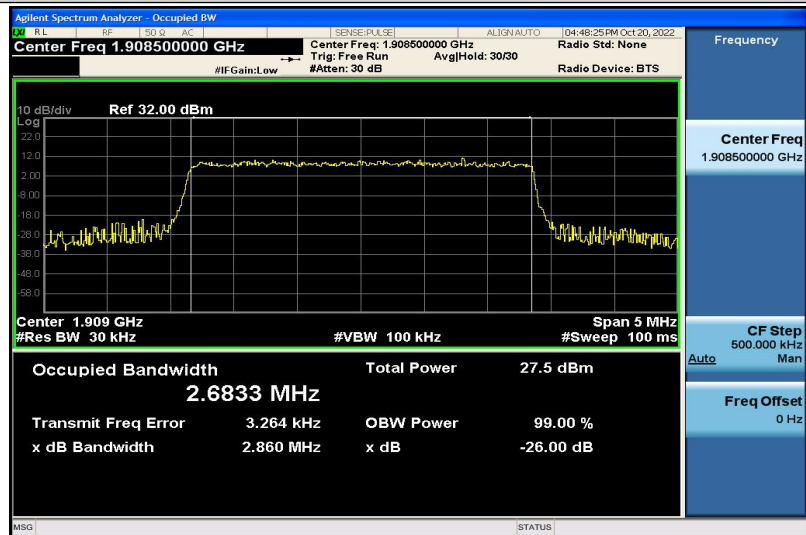
Band2-3MHz-QPSK-19185-15RB#0-2.6833
