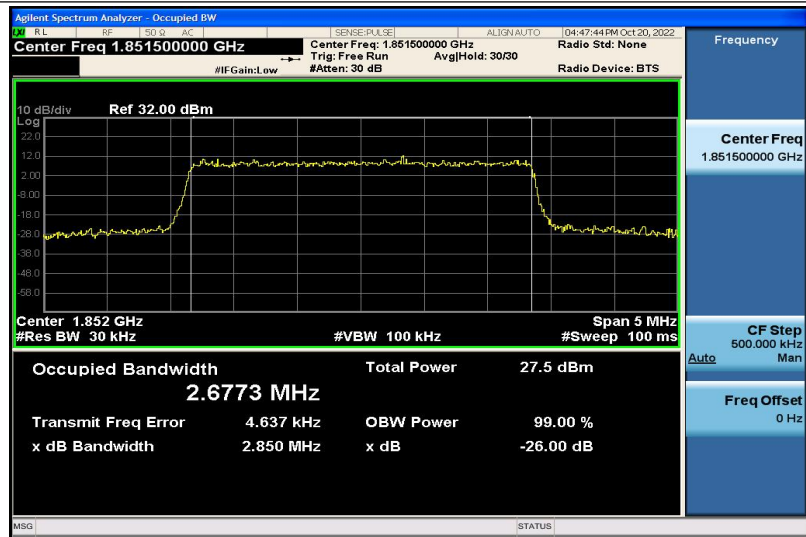
Band2-3MHz-QPSK-18615-15RB#0-2.6773
