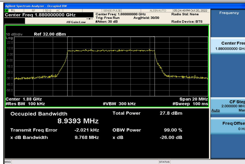
Band2-10MHz-QPSK-18900-50RB#0-8.9393
