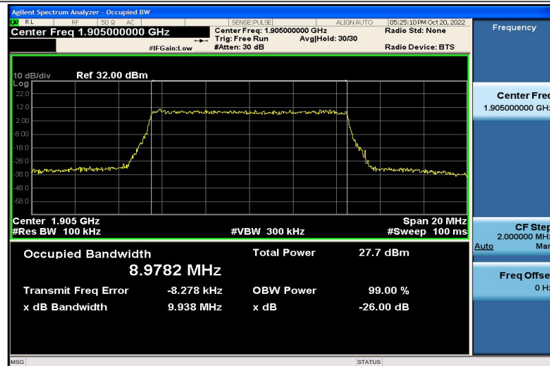
Band2-10MHz-QPSK-19150-50RB#0-8.9782
