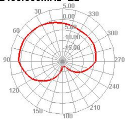
2400.000MHz E2
