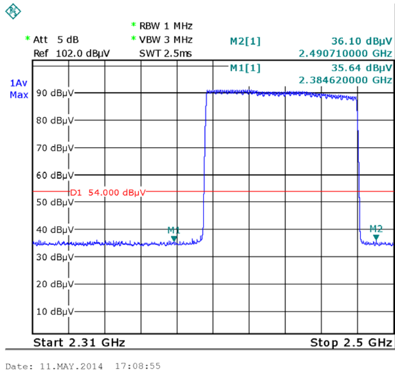
1M-HOPPING-AV
