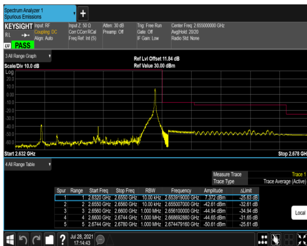
Band41-20MHz-QPSK-41140-1RB#99
