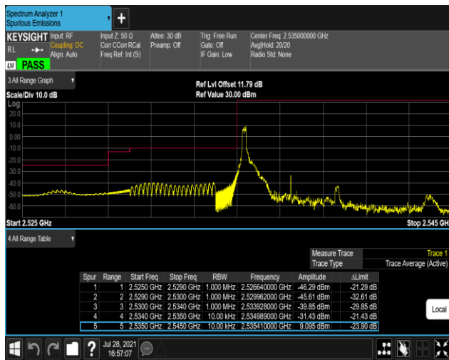
Band41-5MHz-QPSK-40065-25RB#0
