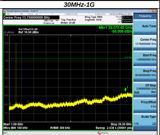
1G-26.5G
