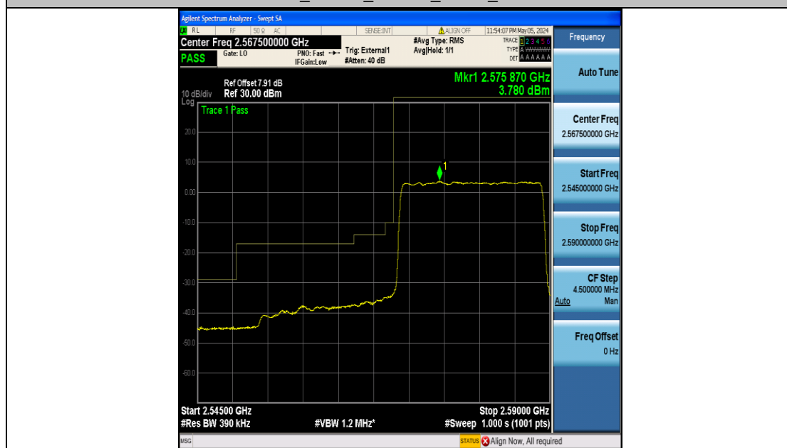
Band38_20MHz_QPSK_37850_100RB#0
