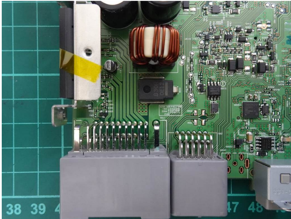
(37) EUT Photo
