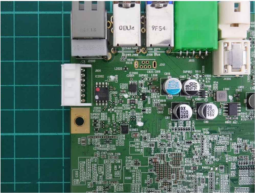
(14) EUT Photo
