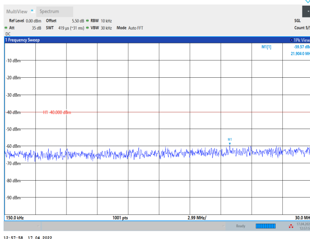
Band30-10MHz-QPSK-27710-1RB#0-Range2:0.15~30MHz
