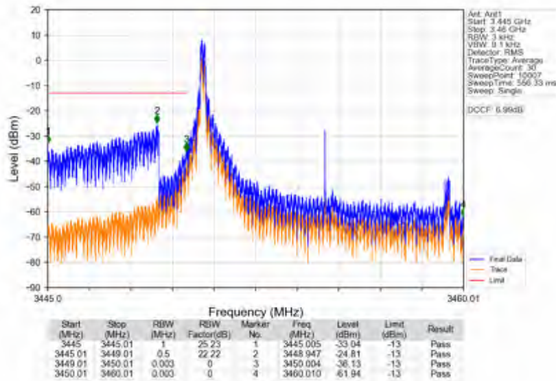
n78e_15kHz_SISO_NTNV_10MHz_DFT-s-OFDM_QPSK_3455.01MHz_Inner_1RB_Left
