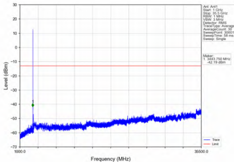
n78e_15kHz_SISO_NTNV_10MHz_DFT-s-OFDM_QPSK_3455.01MHz_Inner_1RB_Left
