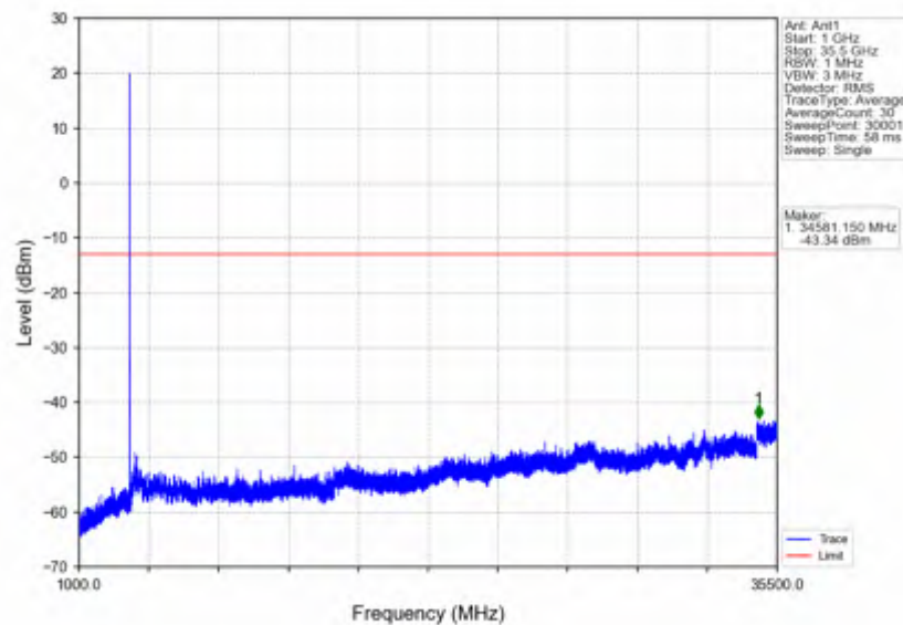
n78e_15kHz_SISO_NTNV_10MHz_CP-OFDM QPSK_3499.995MHz_Edge_1RB_Left
