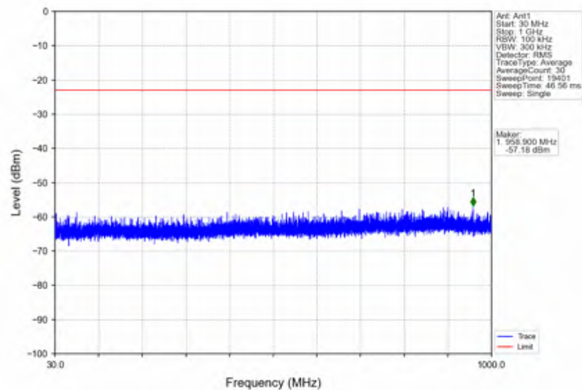
n78e_15kHz_SISO_NTNV_10MHz_CP-OFDM QPSK_3499.995MHz_Edge_1RB_Left
