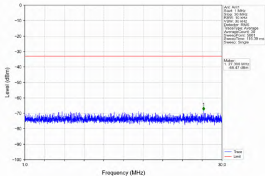
n78e_15kHz_SISO_NTNV_10MHz_CP-OFDM QPSK_3499.995MHz_Edge_1RB_Left
