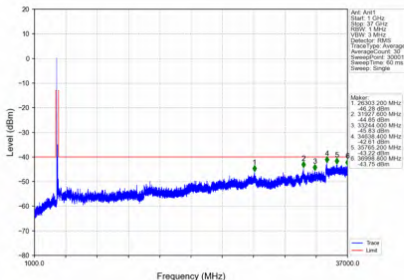
n78d 30kHz SISO NTN 100MHz DFT-s-OFDM QPSK 3600MHz Edge 1RB Left
