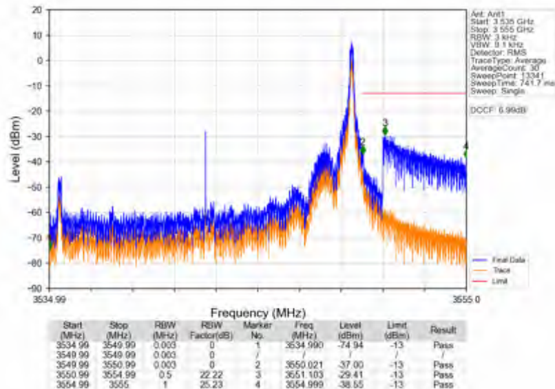
n78e 15kHz SISO NTNV 15MHz DFT-s-OFDM QPSK 3542.49MHz Edge 1RB Right
