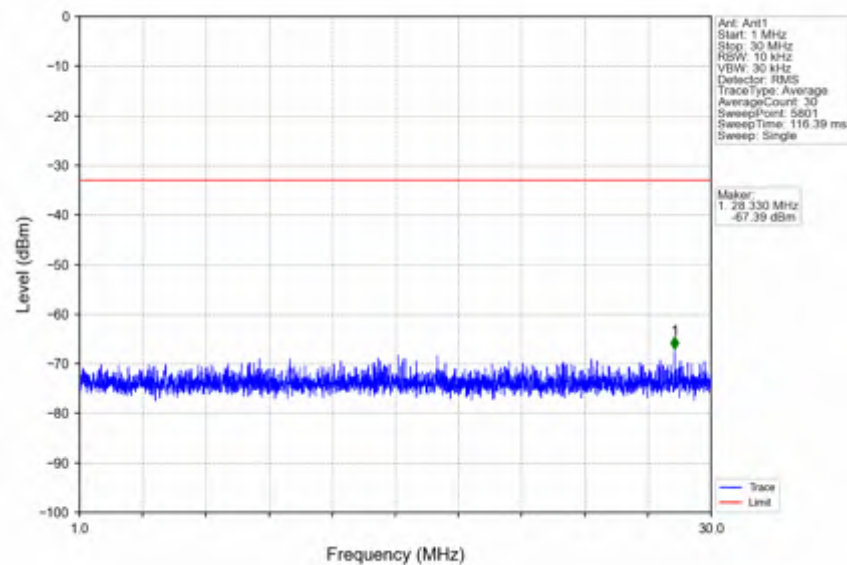
n78e_15kHz_SISO_NTNV_10MHz_DFT-s-OFDM QPSK_3499.995MHz_Edge_1RB_Left
