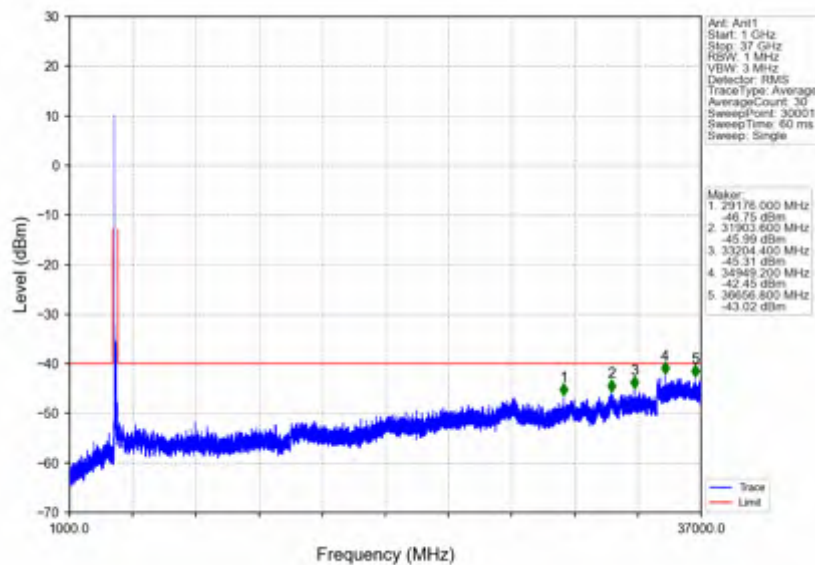
n78d 30kHz SISO NTNv 100MHz CP-OFDM QPSK 3624.99MHz Edge 1RB Left
