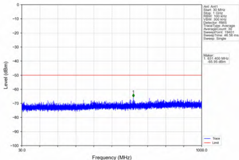
n78d 30kHz SISO NTN 100MHz DFT-s-OFDM QPSK 3600MHz Edge 1RB Left
