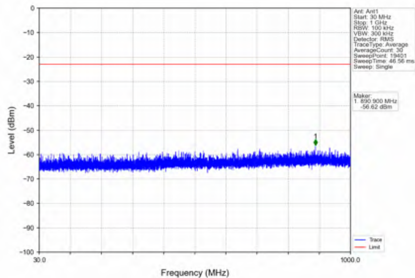
n78e_15kHz_SISO_NTNV_10MHz_DFT-s-OFDM QPSK_3499.995MHz_Edge_1RB_Left
