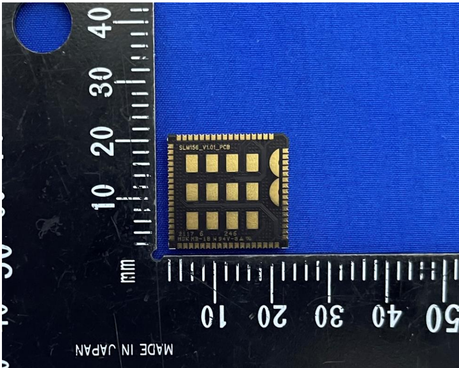
(2) EUT Photo
