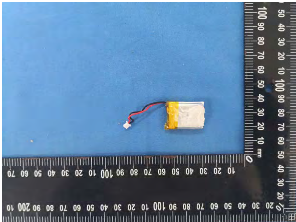
EUT Photo 12 )
