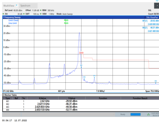
Band38-15MHz-QPSK-38175-1RB#74
