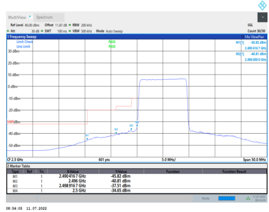
Band7-10MHz-QPSK-20800-50RB#0
