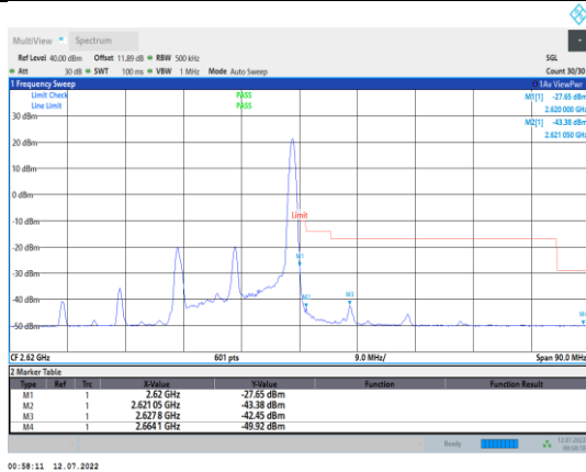
Band38-20MHz-QPSK-38150-1RB#99
