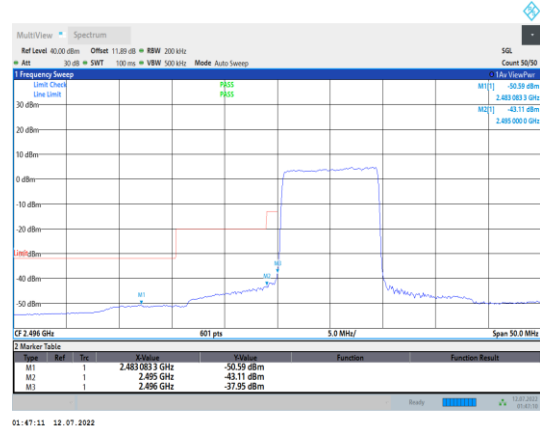
Band41-10MHz-QPSK-39700-50RB#0
