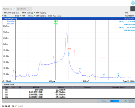
Band41-5MHz-16QAM-41565-1RB#24
