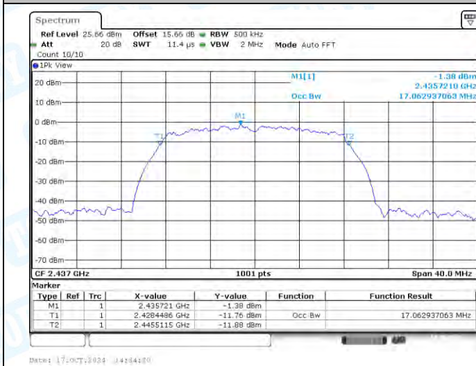
11G-Ant1-2437
