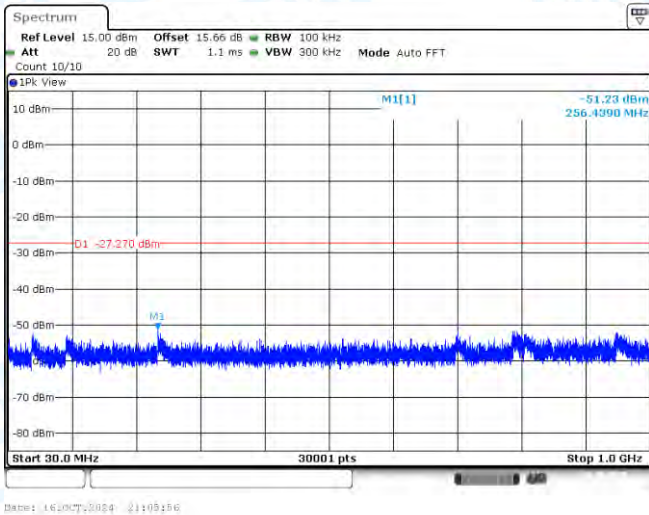
11G-Ant1-2412-30~1000-PASS
