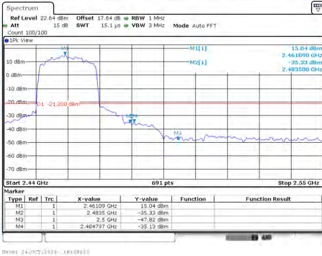
11AX20ISO-Ant1-2462-PASS
