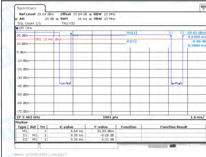
NTVN-11B-Ant1-2462
