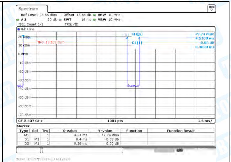
NTVN-11B-Ant1-2437
