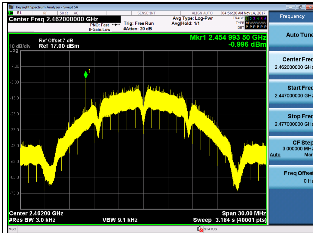
802.11b-2462MHz Chain 0
