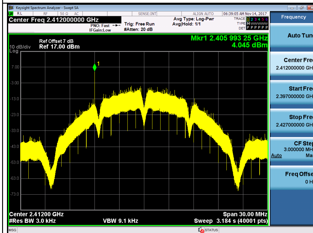
802.11b-2412MHz Chain 1
